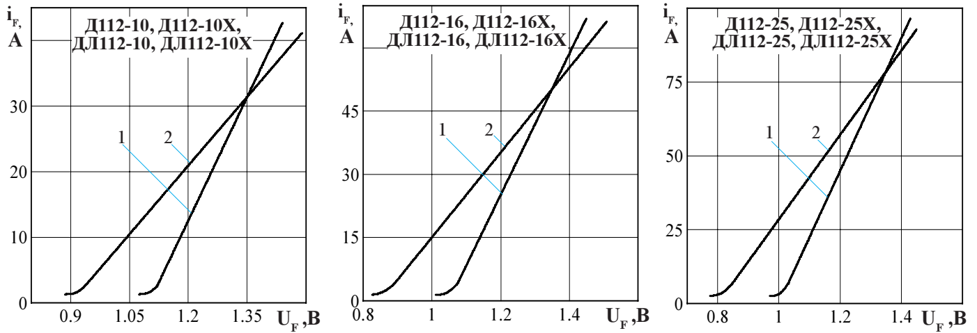
Рисунок 1 - Предельная прямая вольтамперная характеристика при температуре перехода 25^{\circ}\text{C} (1) и максимальной температуре перехода T_{jm} (2) I_F = 3, 14 I_{F(AV)}
