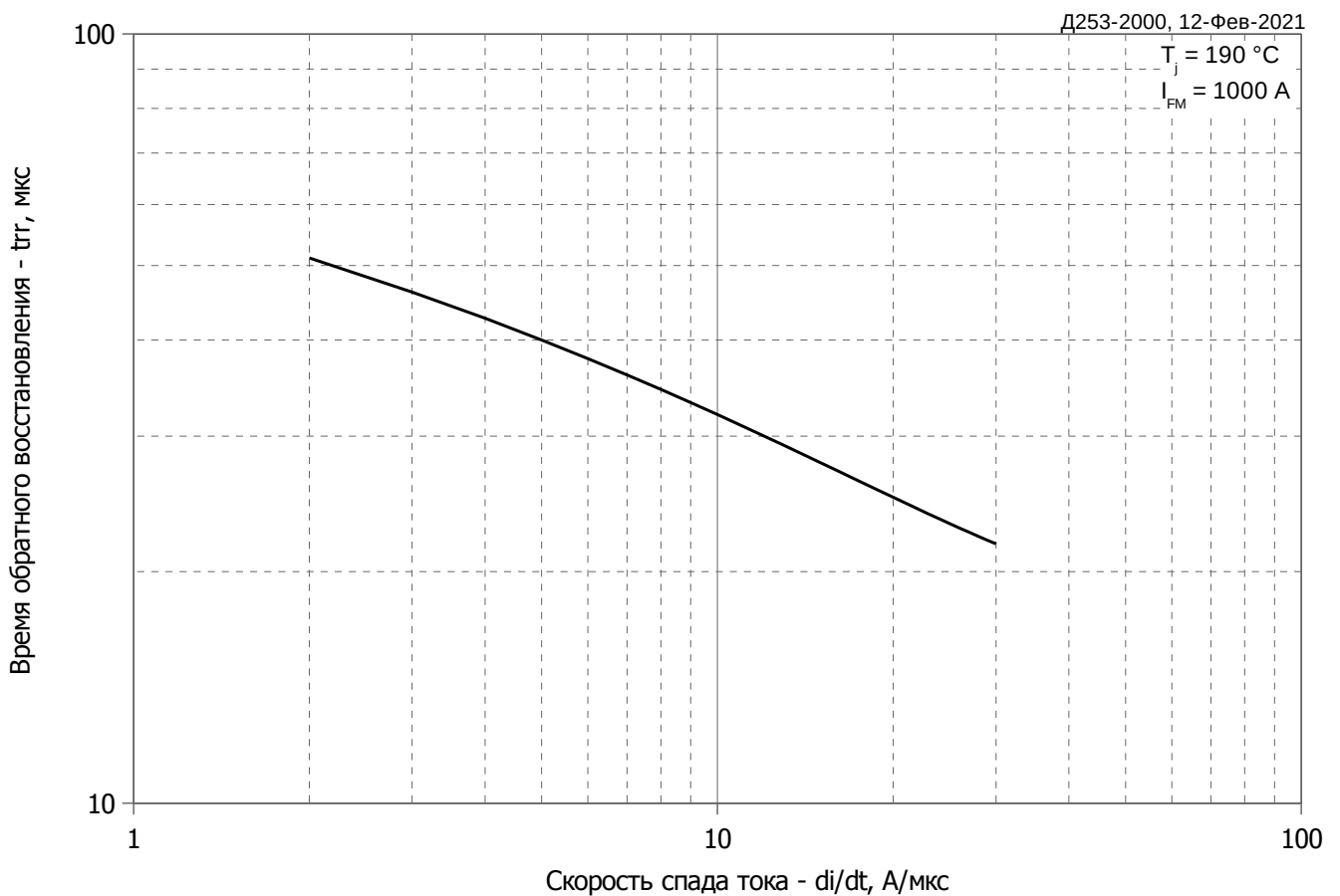
Рис. 6 – Зависимость максимального времени обратного восстановления t_{trr} от скорости спада прямого тока di_R/dt (по ГОСТ 24461, хорда 25%)
