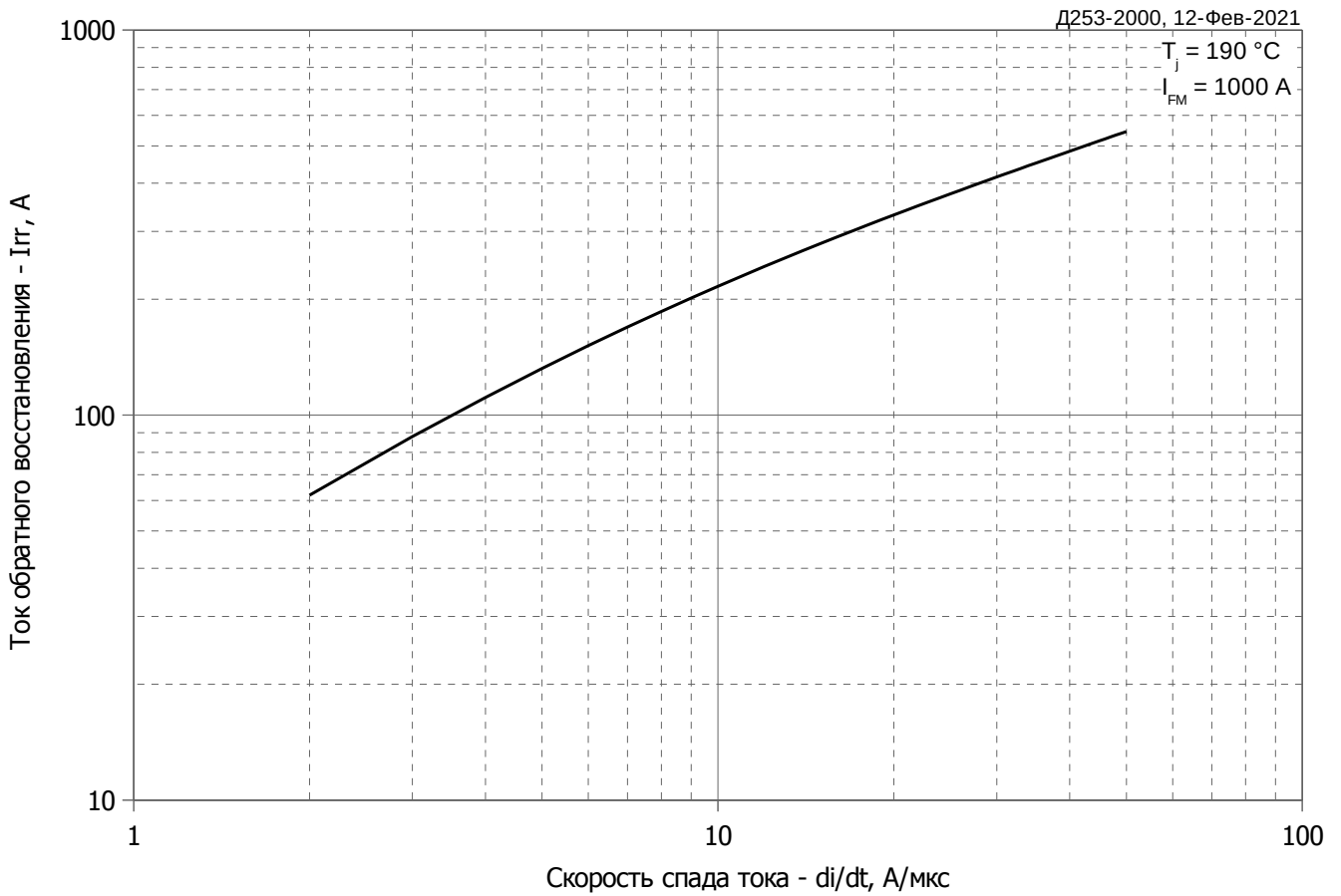
Рис. 5 – Зависимость максимального тока обратного восстановления I_{trr} от скорости спада прямого тока di_R/dt
