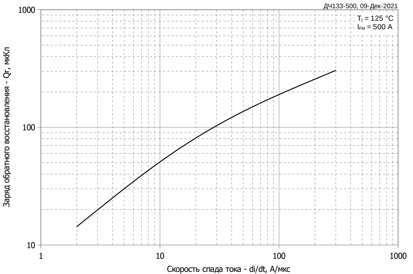
Рис. 4 – Зависимость максимального заряда обратного восстановления Q_g от скорости спада прямого тока di_R/dt (по ГОСТ 24461, хорда 50%)
