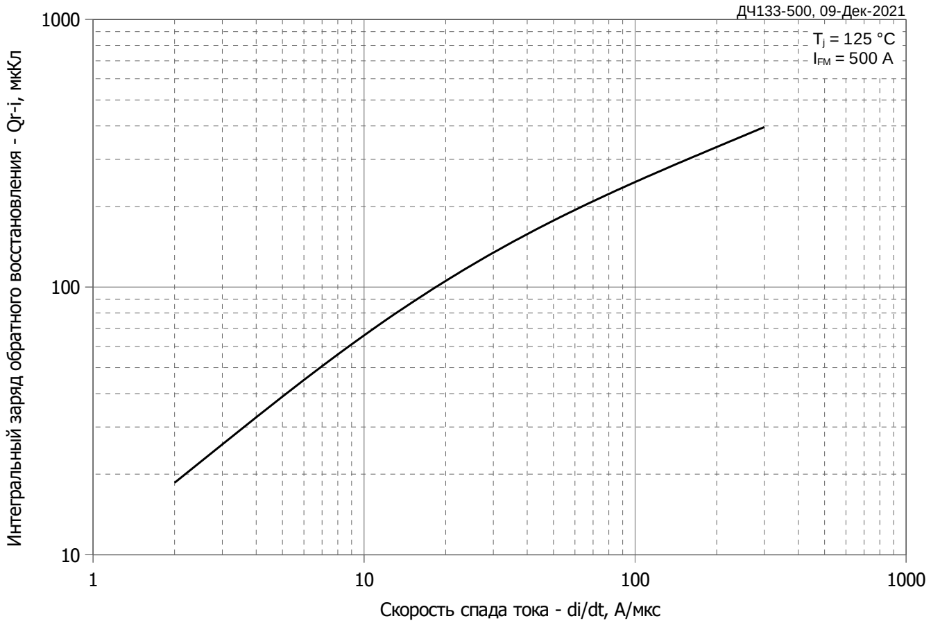
Рис. 3 – Зависимость заряда обратного восстановления Q_{g-i} (интегральный) от скорости спада прямого тока di_R/dt
