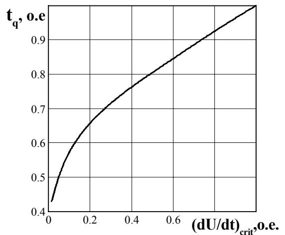
Рисунок 16 - Зависимость времени выключения t_q (о.е.) от скорости нарастания напряжения в открытом состоянии dU_D/dt при T_{im} = 125 \text{ } ^\circ\text{C} ; I_T = I_{T(AV)} ; U_D = 0,67 U_{DRM} ; U_R = 100 \text{ В} ; (di/dt)_f = 5 \text{ A/мкс}
