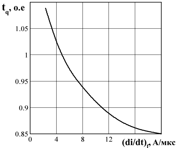
Рисунок 15 - Зависимость времени выключения t_q (о.е.) от скорости спада тока в открытом состоянии (di/dt)_f при T_{jm} = 125^\circ\text{C} ; I_T = I_{T(AV)} ; U_R = 100 В; dU_D/dt = 50 В/мкс; U_D = 0,67 U_{DRM}
