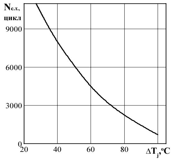
Рисунок 19 - Зависимость максимально допустимого числа циклов N с.т. от перепада температуры перехода ΔT j при циклической токовой нагрузке.
