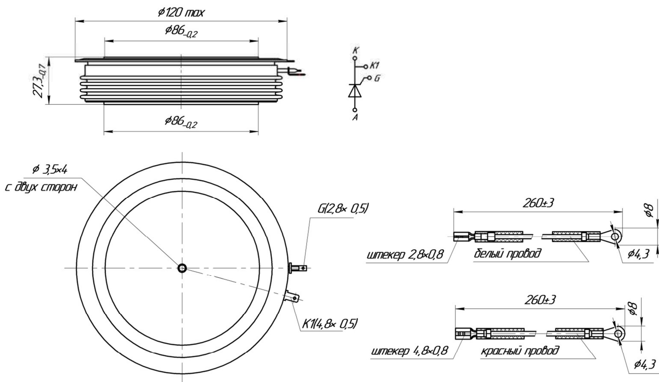
Габаритные и установочные размеры (размеры в мм)
