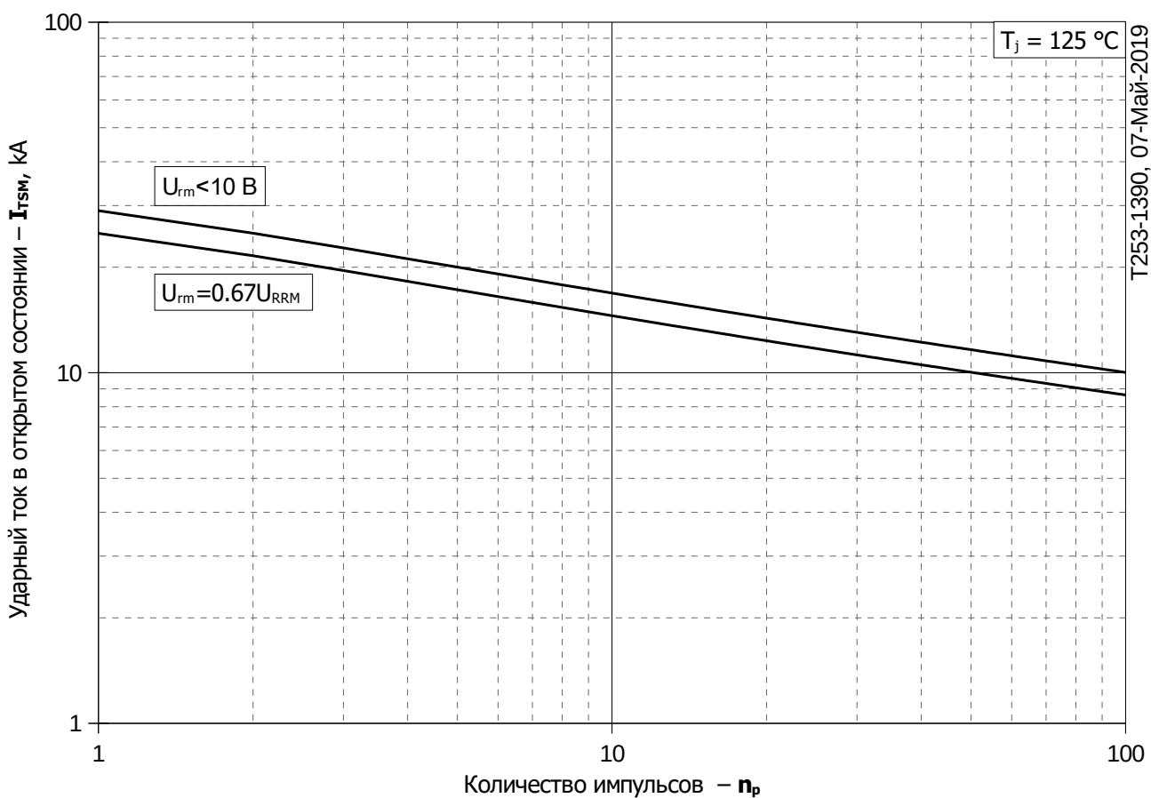
Рис. 14 – Зависимость максимальной амплитуды ударного тока в открытом состоянии I_{TSM} от количества импульсов n_p
