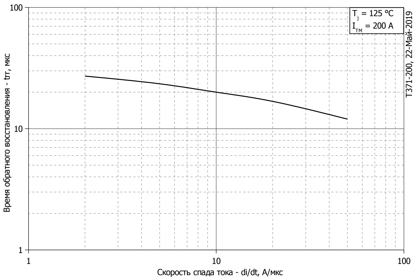
Рис. 6 - Зависимость максимального времени обратного восстановления t тр от скорости спада тока di R /dt (по ГОСТ 24461, хорда 25%) в открытом состоянии
