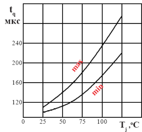
Рисунок 12 - Зависимость времени выключения t_q от температуры структуры T_j при I_T = I_{TAVM} ; U_D = 0,67 U_{DRM} ; U_R = 100 В; (di/dt)_f = 5 А/мкс; dU_D/dt = 50 В/мкс
