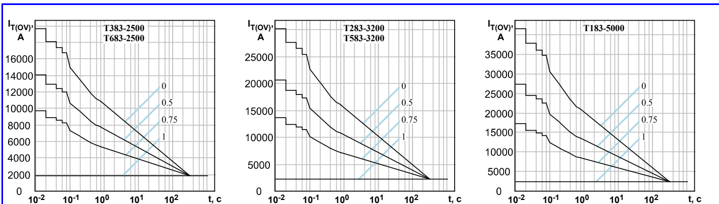
Рисунок 11: Зависимость допустимой амплитуды тока перегрузки в открытом состоянии I_{T(OV)} синусоидальной формы частотой 50 Гц от длительности перегрузки t при температуре окружающей среды 40^\circ\text{C} и при различных значениях k , равных отношению предшествующего перегрузке тока I_T к допустимому среднему току в открытом состоянии I_{T(AV)} на охладителе О193.
