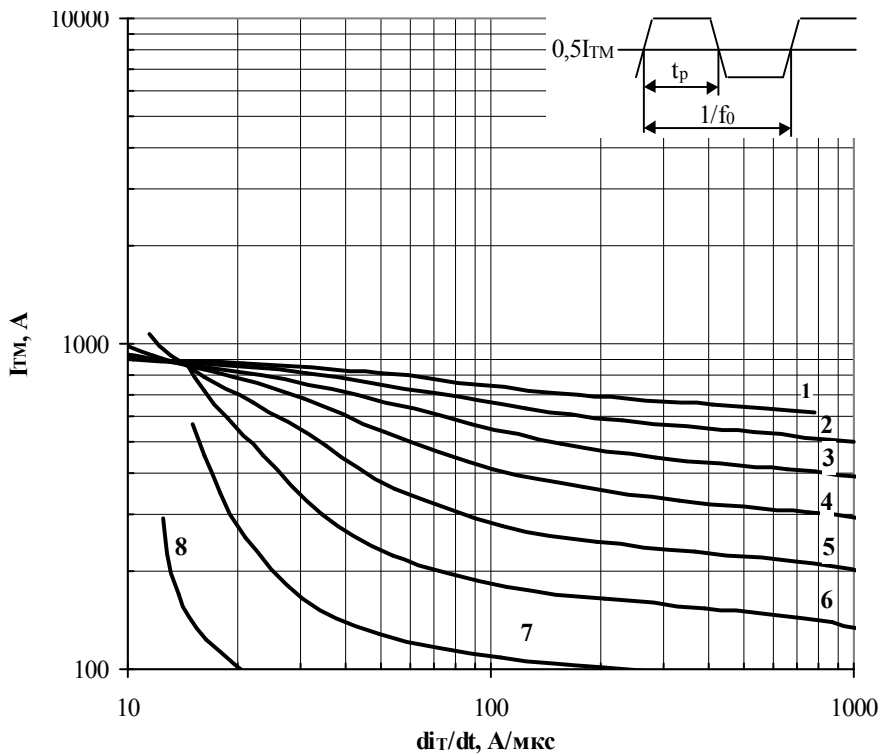
Рис. 10 – Зависимость импульсного тока в открытом состоянии I_{TM} трапецевидной формы тока от скорости нарастания прямого тока di_T/dt , длительности импульсов t_p=1/2f_0 и температуры корпуса T_c=65\text{ }^\circ\text{C} .
