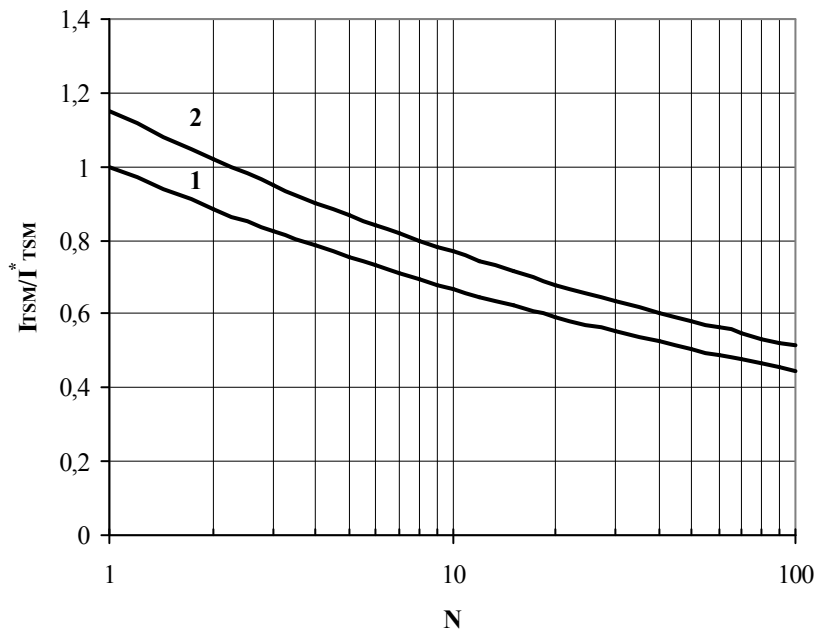
Рис. 30 – Ударный ток I_{TSM} от количества полусинусоидальных импульсов тока длительностью 10 мс 1 – T_j = 125^\circ C 2 – T_j = 25^\circ C
