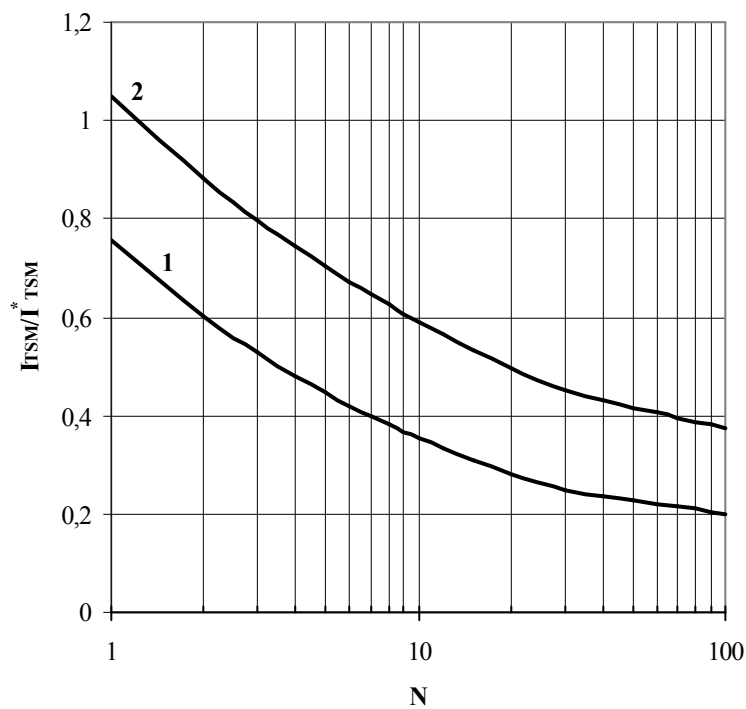
Рис. 31 – Ударный ток I_{TSM} от количества полусинусоидальных импульсов тока длительностью 10 мс 1 – T_j = 125^\circ C 2 – T_j = 25^\circ C
