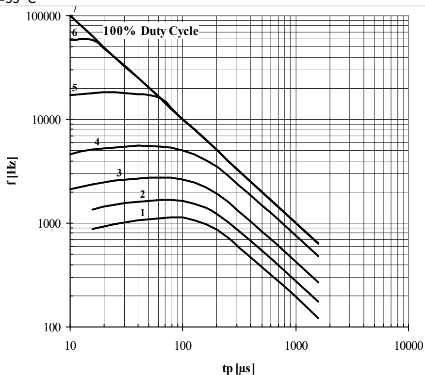
Рис. 11 — Зависимость частоты синусоидальных импульсов тока от длительности импульсов тока
