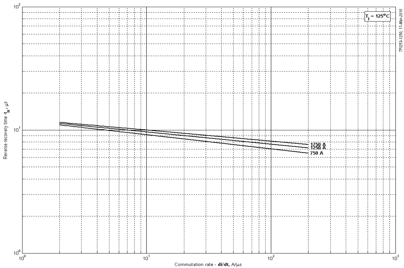
Рис. 6 – Максимальное время обратного восстановления, t_{tr} (по ГОСТ 24461, хорда 50%)
