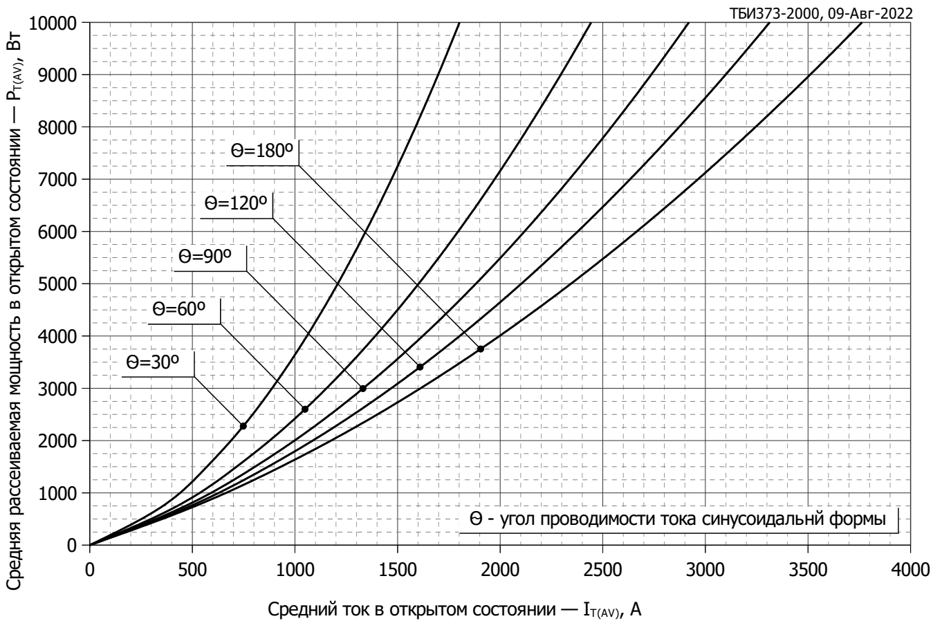
Рис. 28 - Зависимость потерь мощности P_{T(AV)} от среднего тока в открытом состоянии I_{T(AV)} синусоидальной формы при различных углах проводимости ( f=50 \text{ Гц} )
