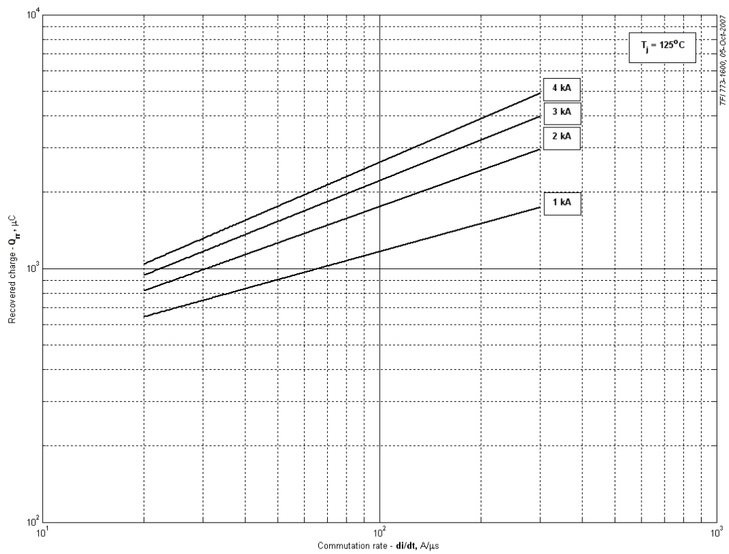
Рис. 4 – Максимальный заряд обратного восстановления, Q_{rr} (по ГОСТ 24461, хорда 50%)
