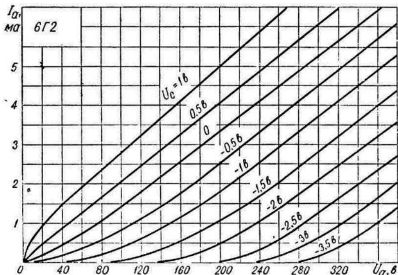
Рис. 1 Усредненные характеристики зависимости тока анода от напряжения на аноде.
