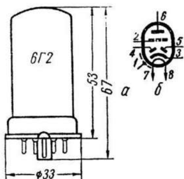
Рис. 177. Лампа 6Г2.
