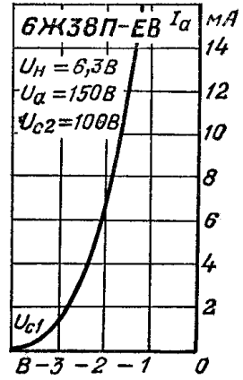
Анодно-сеточная характеристика.
