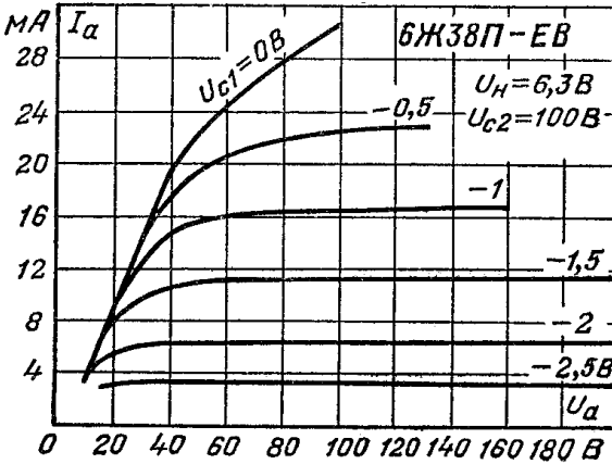
Анодные характеристики.
