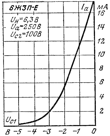
Анодно-сеточная характеристика.
