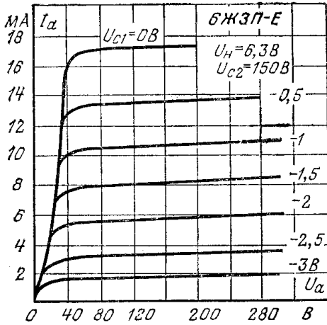
Анодные характеристики.
