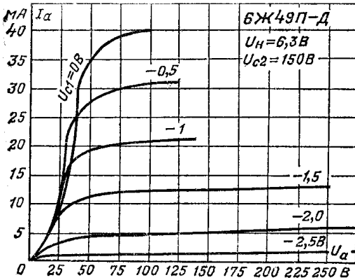
Анодные характеристики.
