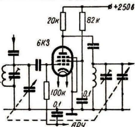
Рис. 295. Схема применения лампы 6K3 в усилителе высокой частоты.
