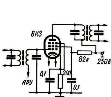
Рис. 294. Схема применения лампы 6K3 в каскаде усиления напряжения промежуточной частоты.
