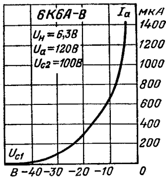
Анодно-сеточная характеристика (начальный участок).
