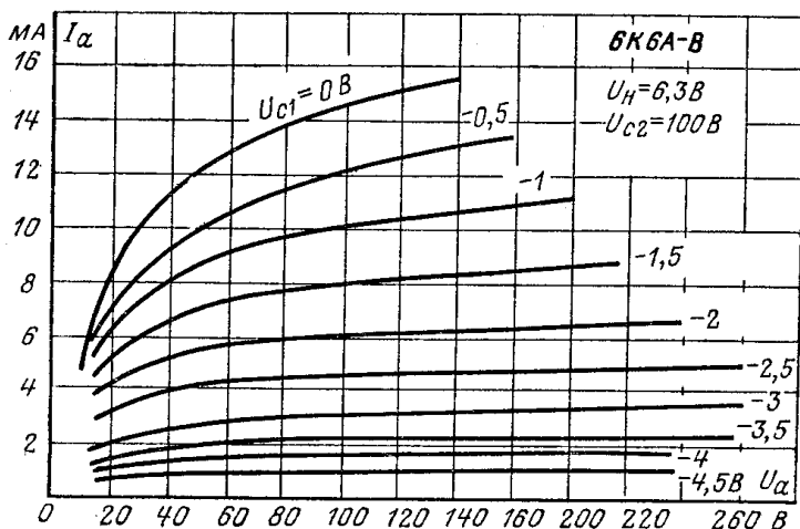
Анодные характеристики.
