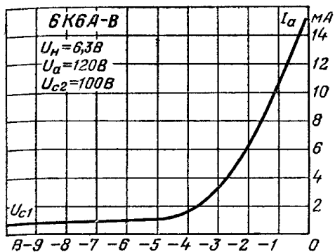
Анодно-сеточная характеристика.
