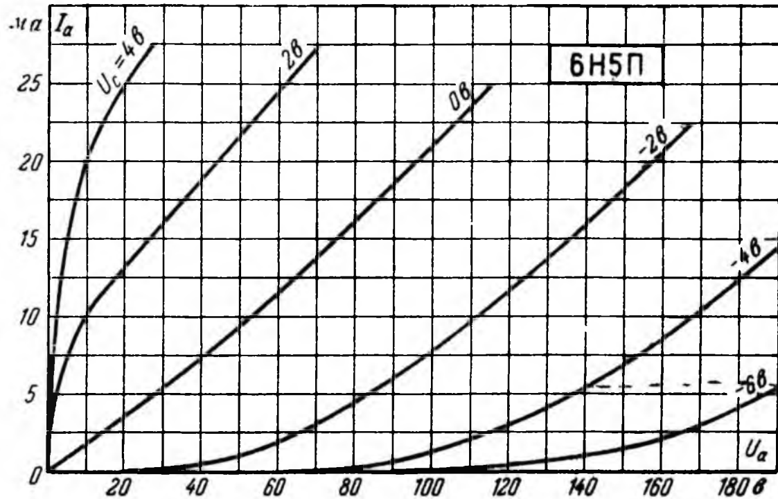
Анодные характеристики лампы 6Н5П (для каждого триода).
