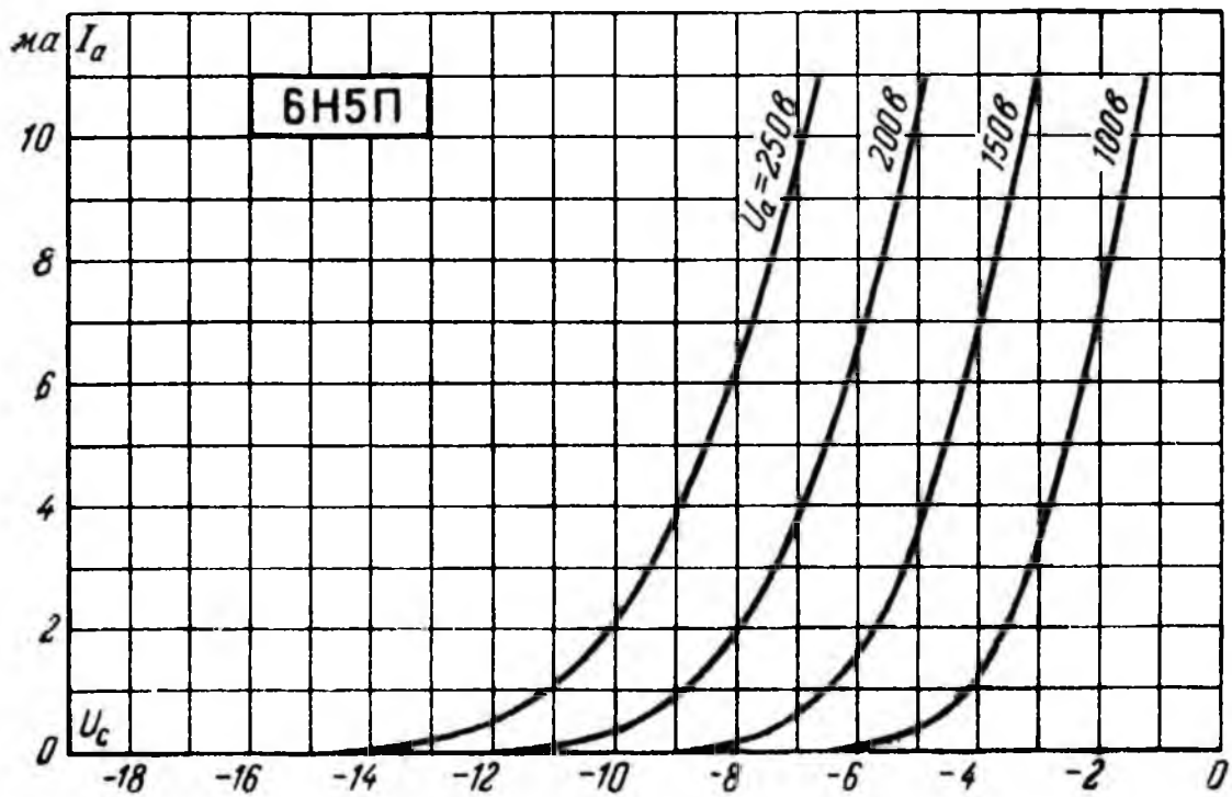
Анодно-сеточные характеристики лампы 6Н5П (для каждого триода).
