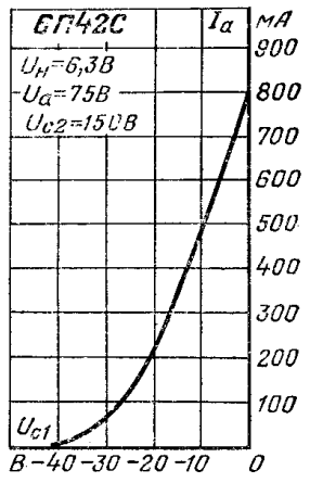
Анодно-сеточная характеристика.
