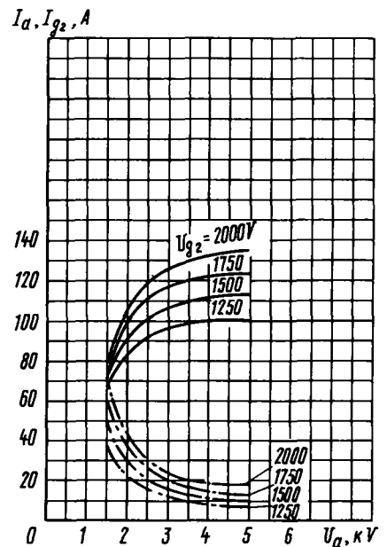
Усредненные характеристики: избыточное напряжение сетки первой ( U_{g1} ) в импульсе равно 150 В; — анодные; --- сеточно-анодные (по сетке первой)
