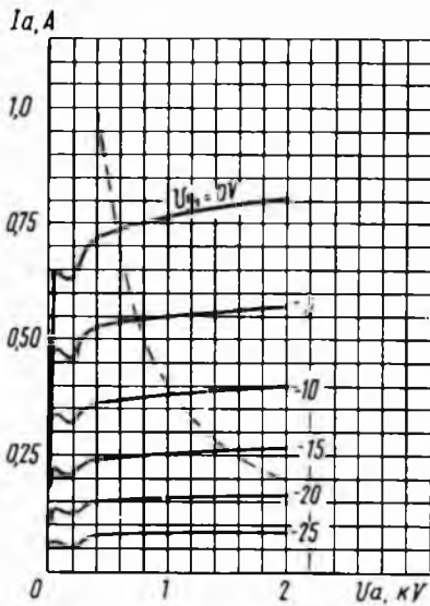
Усредненные анодные характеристики: U_1 = 6.3 \text{ В}; U_{g2} = 275 \text{ В}; — ток анода ( I_a ); - - - - наибольшая мощность, рассеиваемая анодом ( P_{a \text{ макс}} ) Averaged Anode Characteristic Curves: U_1 = 6.3 \text{ V}; U_{g2} = 275 \text{ V}; — I_a ; - - - - P_{a \text{ макс}}
