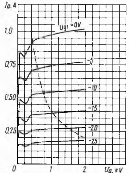
Усредненные анодные характеристики: U_1 = 6.3 \text{ В}; U_{g2} = 325 \text{ В}; — ток анода ( I_a ); - - - - наибольшая мощность, рассеиваемая анодом ( P_{a \text{ макс}} ) Averaged Anode Characteristic Curves: U_1 = 6.3 \text{ V}; U_{g2} = 325 \text{ V}; — I_a ; - - - - P_{a \text{ макс}}
