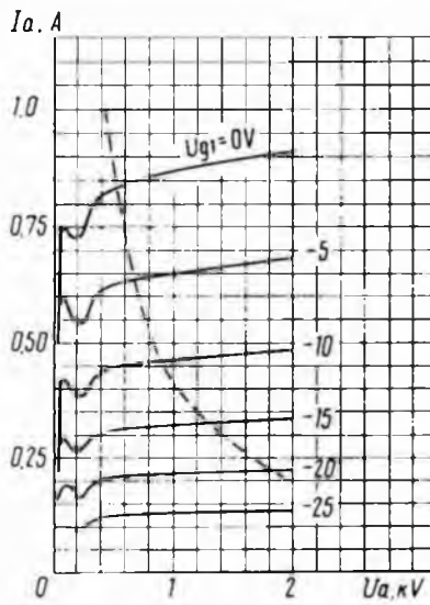
Усредненные анодные характеристики: U_1 = 6.3 \text{ В}; U_{g2} = 300 \text{ В}; — ток анода ( I_a ); - - - - наибольшая мощность, рассеиваемая анодом ( P_{a \text{ макс}} ) Averaged Anode Characteristic Curves: U_1 = 6.3 \text{ V}; U_{g2} = 300 \text{ V}; — I_a ; - - - - P_{a \text{ макс}}
