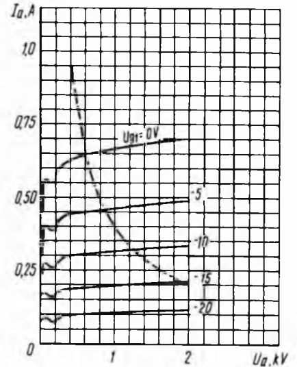
Усредненные анодные характеристики: U_1 = 6.3 \text{ В}; U_{g2} = 250 \text{ В}; — ток анода ( I_a ); - - - - наибольшая мощность, рассеиваемая анодом ( P_{a \text{ макс}} ) Averaged Anode Characteristic Curves: U_1 = 6.3 \text{ V}; U_{g2} = 250 \text{ V}; — I_a ; - - - - P_{a \text{ макс}}
