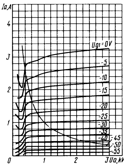
Усредненные анодные характеристики: U_1 = 12,6 \text{ В}; U_{g2} = 350 \text{ В}; — — — наибольшая мощность, рассеиваемая анодом ( P_{a \text{ max}} ) Averaged Anode Characteristic Curves: U_1 = 12.6 \text{ V}; U_{g2} = 350 \text{ V}; — — — P_{a \text{ max}}
