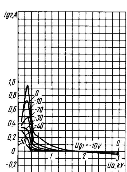
Усредненные сеточно-анодные характеристики (по сетке второй): U_1 = 12,6 \text{ В}; U_{g2} = 350 \text{ В} Averaged Grid 2-Anode Characteristic Curves: U_1 = 12.6 \text{ V}; U_{g2} = 350 \text{ V}
