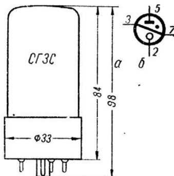
Рис. 619. Стабилитрон СГЗС: а — основные размеры; б — схематическое изображение цоколя; 2 — катод; 3 и 4 — перемычка; 5 — анод.
