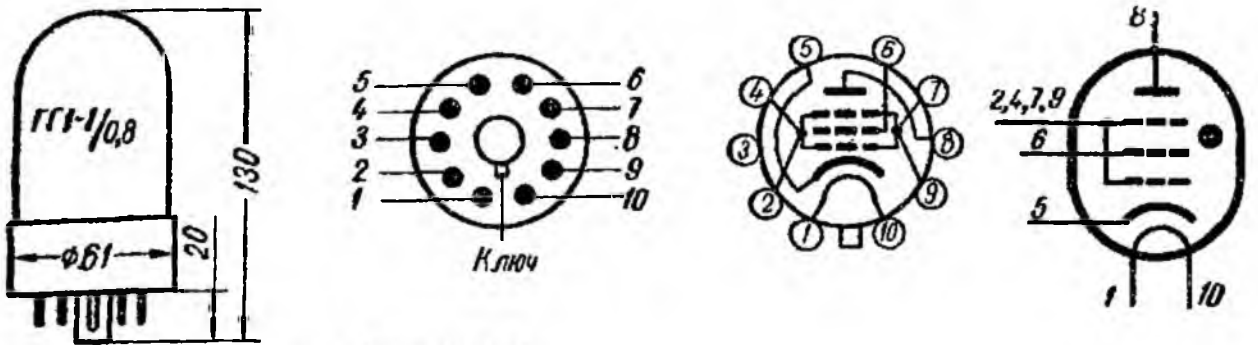
Рис. 28. Тиратрон ТГ1-1/0,8:
