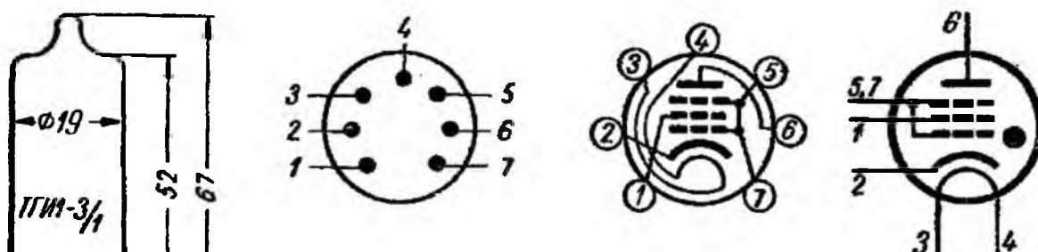
Рис. 44. Тиратрон ТГИ1-3/1:
