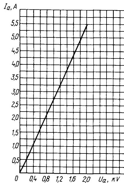
Усредненная импульсная анодная характеристика: U_i = 5 В Averaged Peak Anode Characteristic Curve: U_i = 5 V
