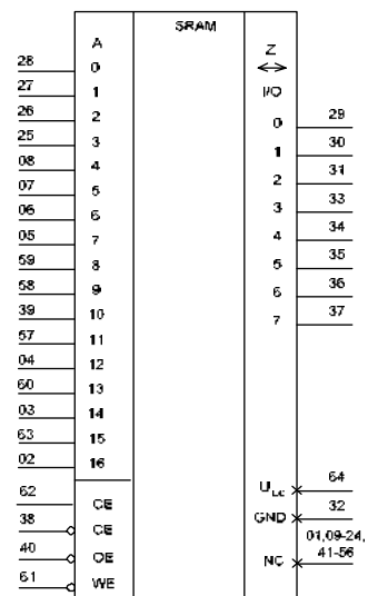
Рисунок 1 – Условное графическое обозначение микросхем 1635PY3Y
