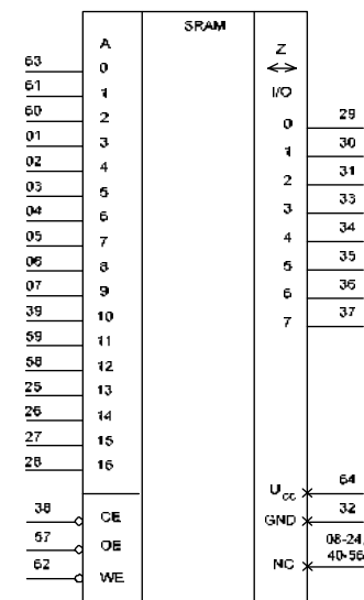
Рисунок 2 – Условное графическое обозначение микросхем 1635PY3AY
