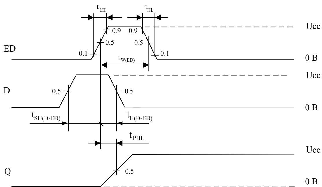
Временная диаграмма работы микросхемы
