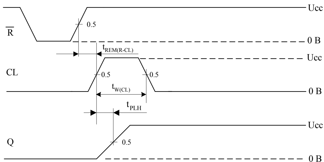
Рисунок 1 – Временная диаграмма входных и выходных импульсов при контроле динамических параметров микросхемы
