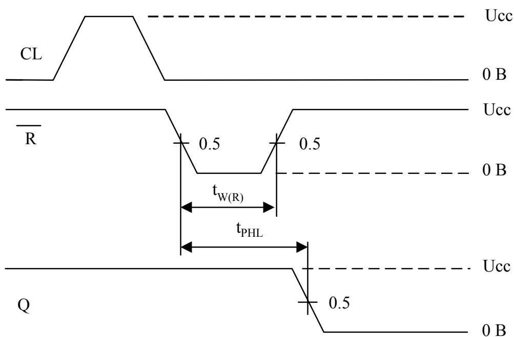
Рисунок 2 – Временная диаграмма входных и выходных импульсов при контроле динамических параметров микросхемы
