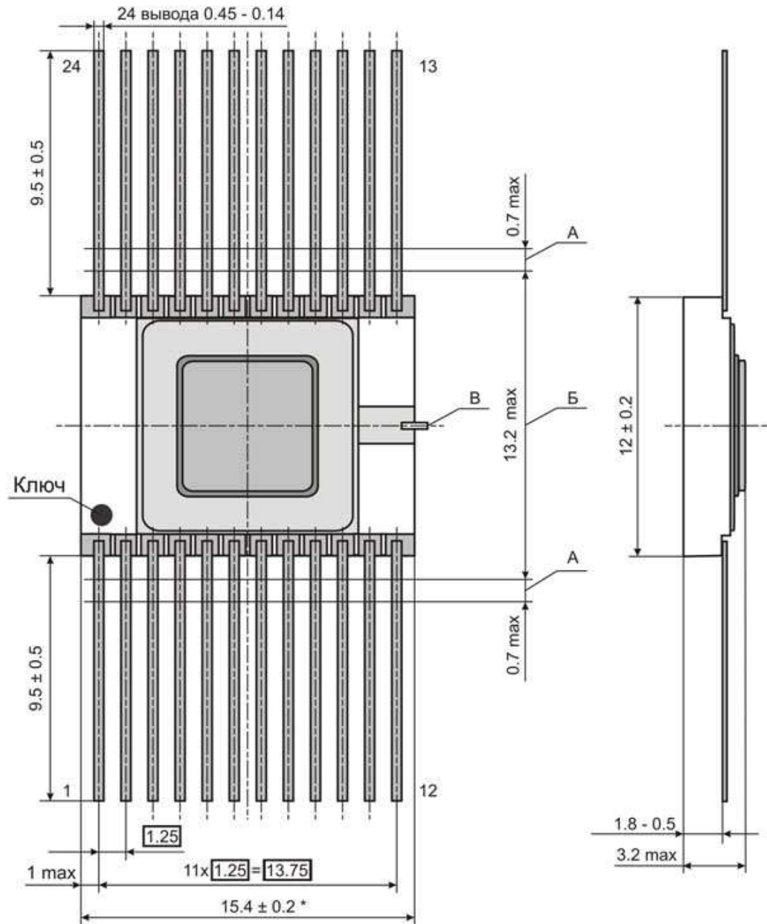
Рис.2. Корпус 4118.24-2.01 размеры в миллиметрах.
