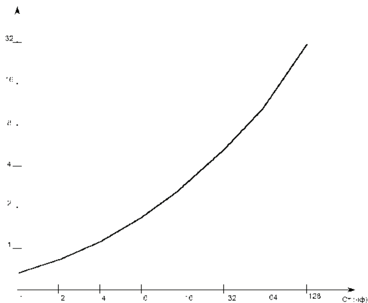
Рисунок 3 – Зависимость «мертвого» времени t от емкости время-задающего конденсатора C_2 (согласно типовой схеме включения).
