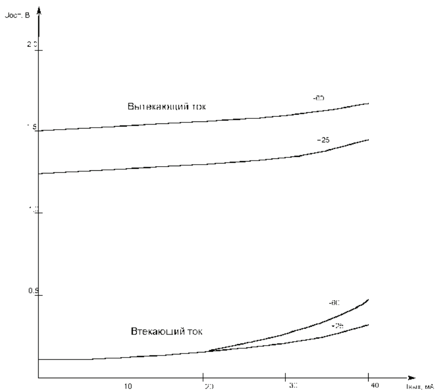
Рисунок 7 – Зависимости остаточного напряжения выходного каскада U_{ост} от втекающего и вытекающего выходных токов I_{вых}
