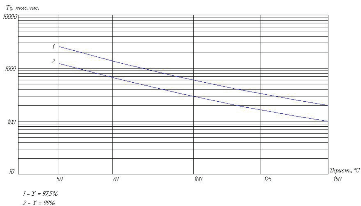
Рисунок 9 – Зависимость гамма–процентной наработки до отказа T_\gamma микросхем от температуры кристалла T_{кр}
