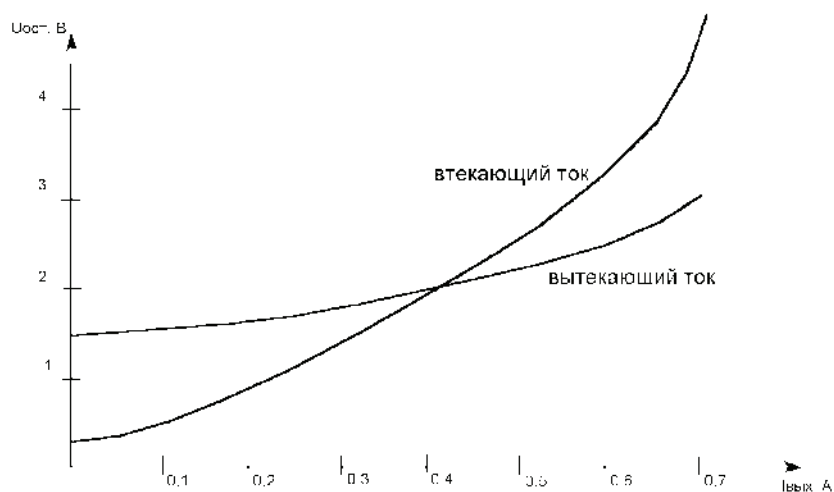
Рисунок 6 – Зависимость остаточного напряжения U_{ост} выходного каскада от втекающего и вытекающего выходных токов I_{вых} (по переменному току).
