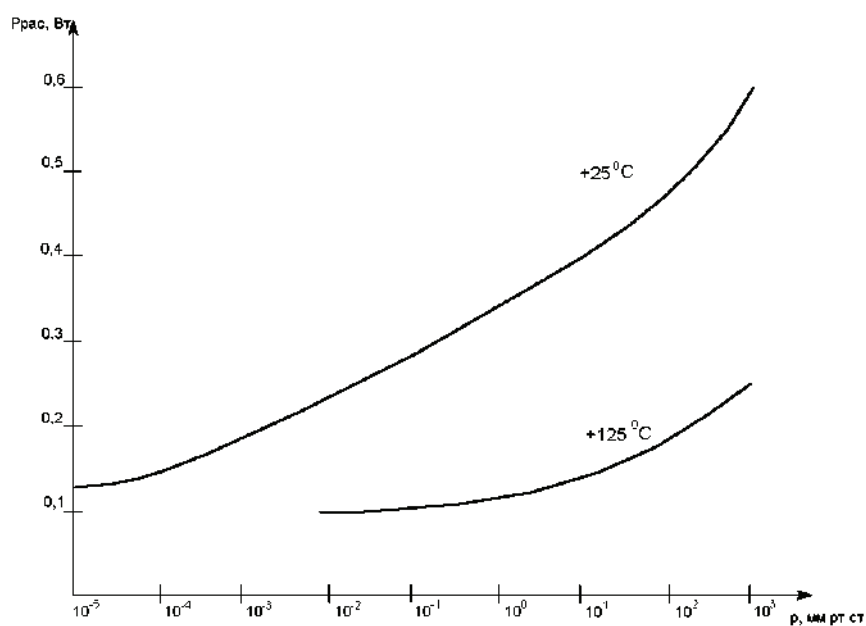
Рисунок 2 – Зависимость рассеиваемой мощности P_{\text{рас}} от атмосферного давления P при заданной температуре окружающей среды T_{\text{окр}}
