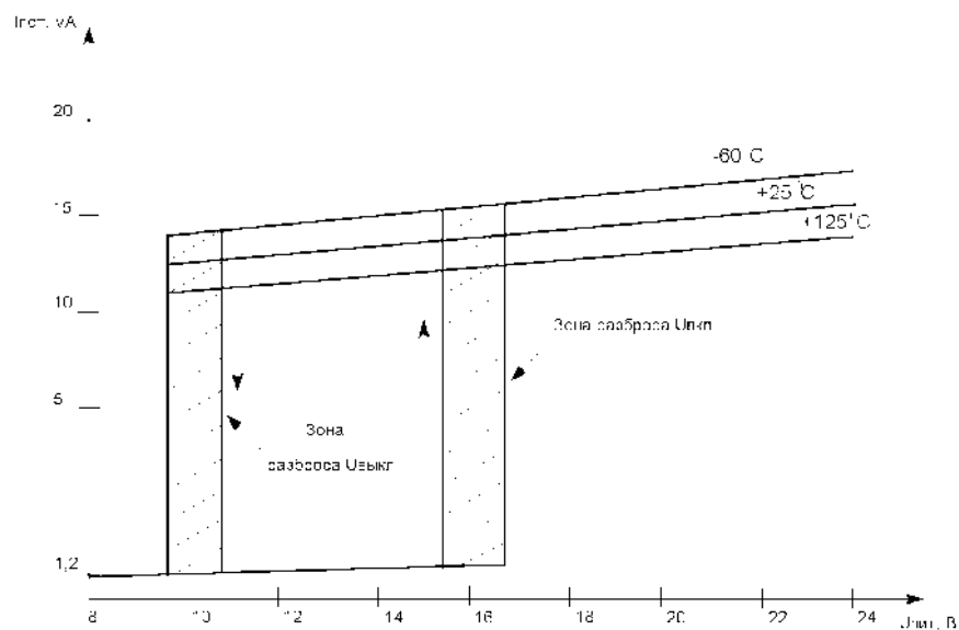
Рисунок 5 – Зависимость тока потребления I_{\text{Пот}} от напряжения питания U_{\text{Пит}} для микросхемы 1114EY7UIM, 1114EY9UIM
