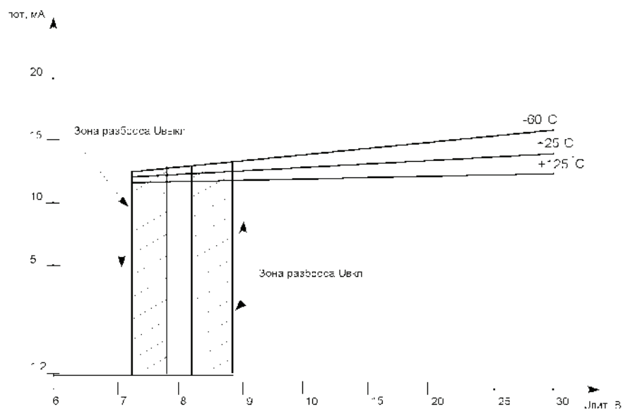
Рисунок 4 – Зависимость тока потребления I_{\text{Пот}} от напряжения питания U_{\text{Пит}} для микросхемы 1114EY8UIM, 1114EY10UIM
