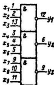
Условное графическое обозначение К136ЛА4
