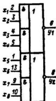
Условное графическое обозначение К136ЛР1
