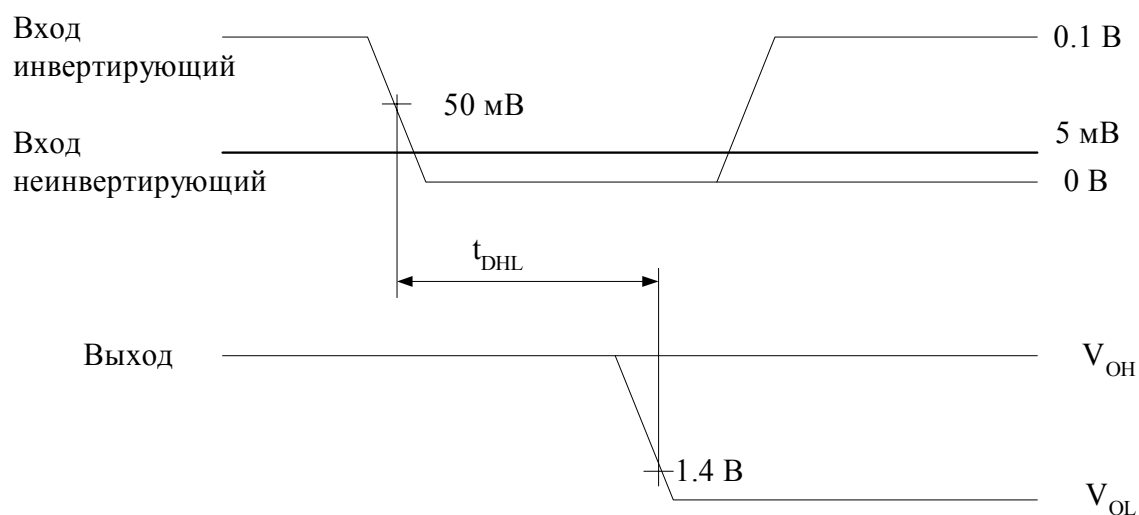
Рисунок 1 – Временная диаграмма
