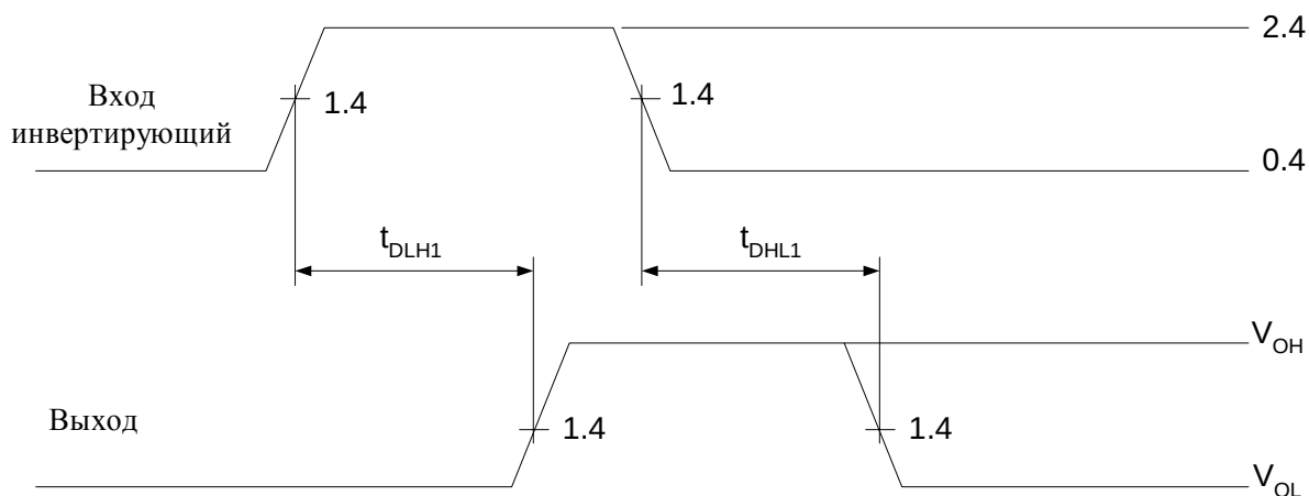
Рисунок 1 – Временная диаграмма
