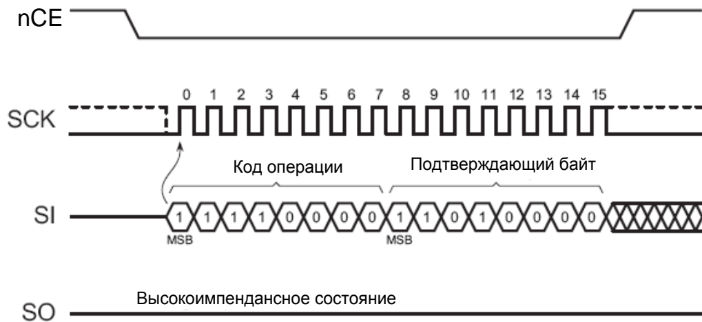
Рисунок 26 – Операция сброса
