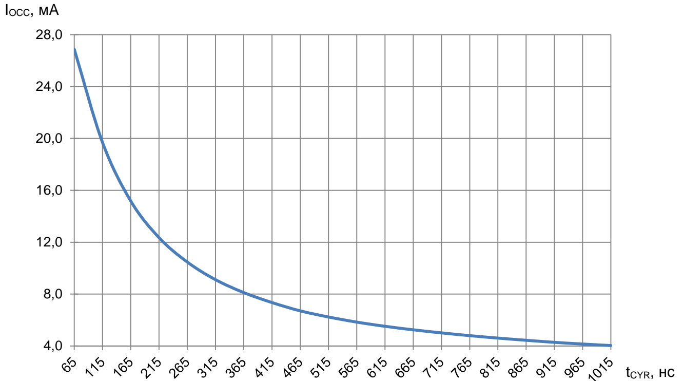
Рисунок 44 – Зависимость динамического тока потребления от времени цикла считывания информации при U_{CC} = 3,6 В и T = 25 °C
