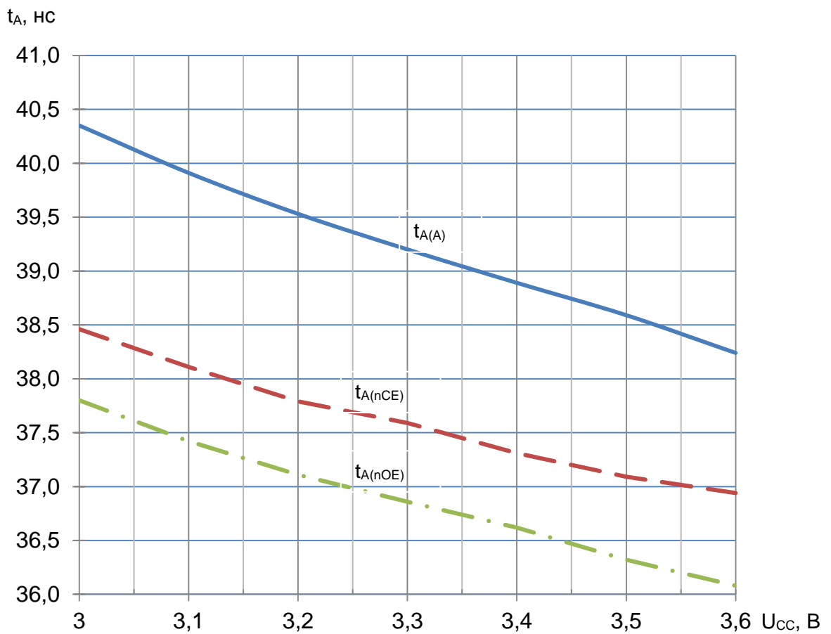
Рисунок 46 – Зависимость времени выборки адреса, t_{A(A)} , времени выборки по сигналу nCE, t_{A(CE)} , времени выборки по сигналу nOE, t_{A(OE)} от напряжения питания при T = 125 °С
