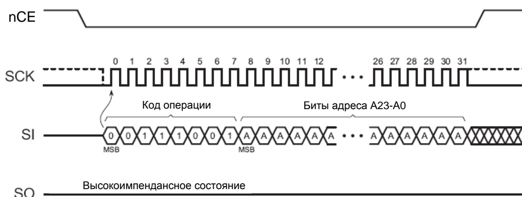
Рисунок 22 – Операция снятия защиты сектора
