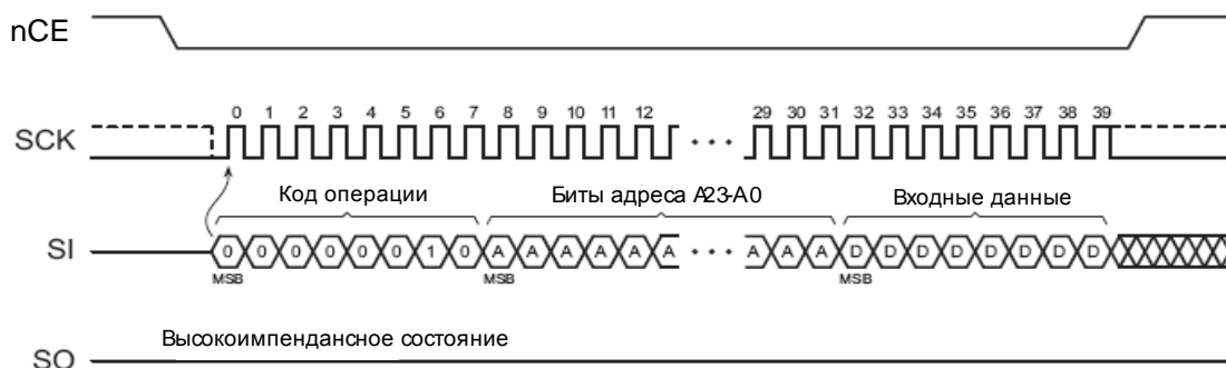
Рисунок 16 – Операция программирования байта
