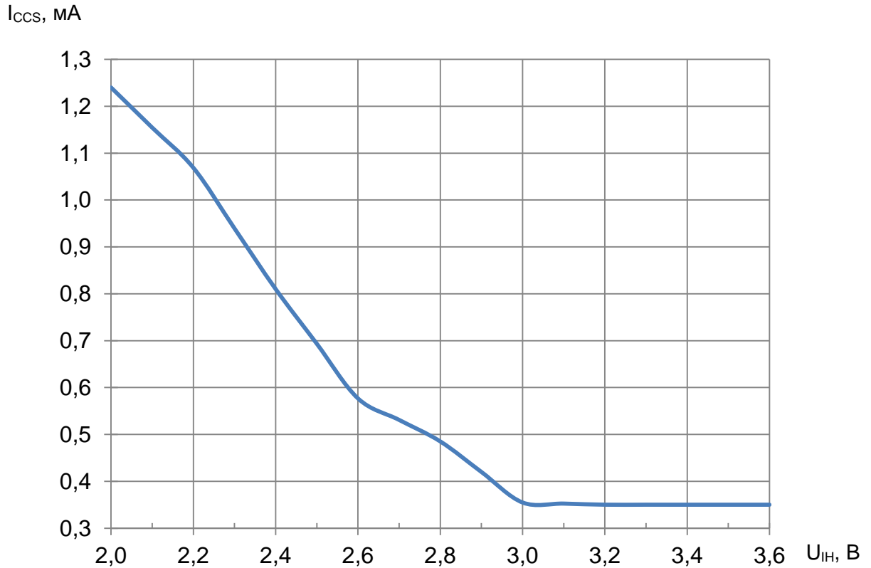
Рисунок 39 – Зависимость тока потребления в режиме хранения от входного напряжения высокого уровня при U_{CC} = 3,6 В, U_{IL} = 0 В, f = 0 МГц, T = 25 °С
