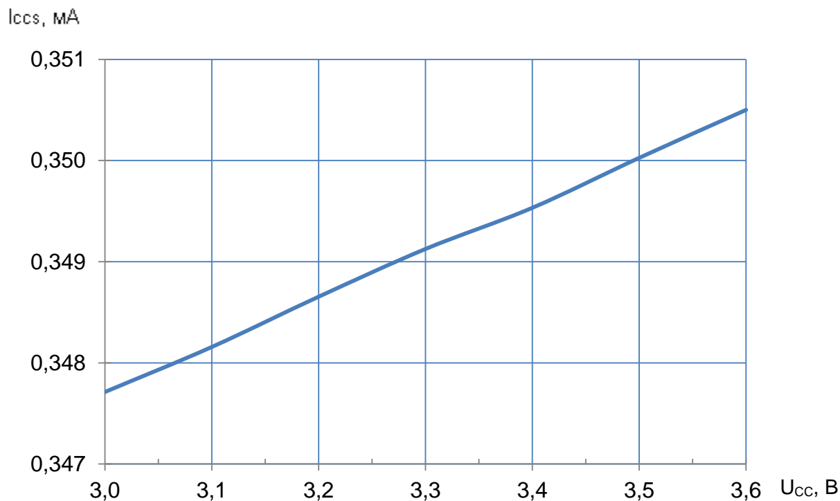
Рисунок 37 – Зависимость тока потребления в режиме хранения от напряжения питания при T = 25\text{ °C}
