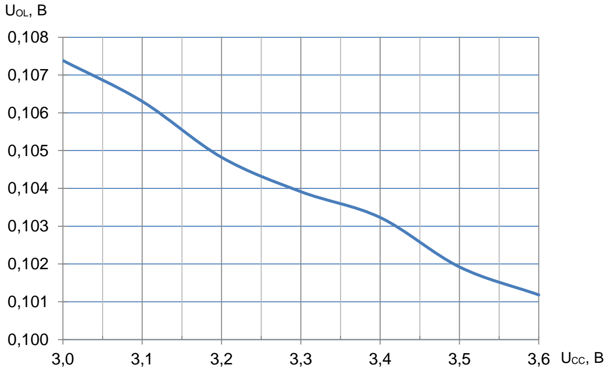
Рисунок 41 – Зависимость выходного напряжения низкого уровня от напряжения питания при I_{OL} = 4 мА, T = 25 °С
