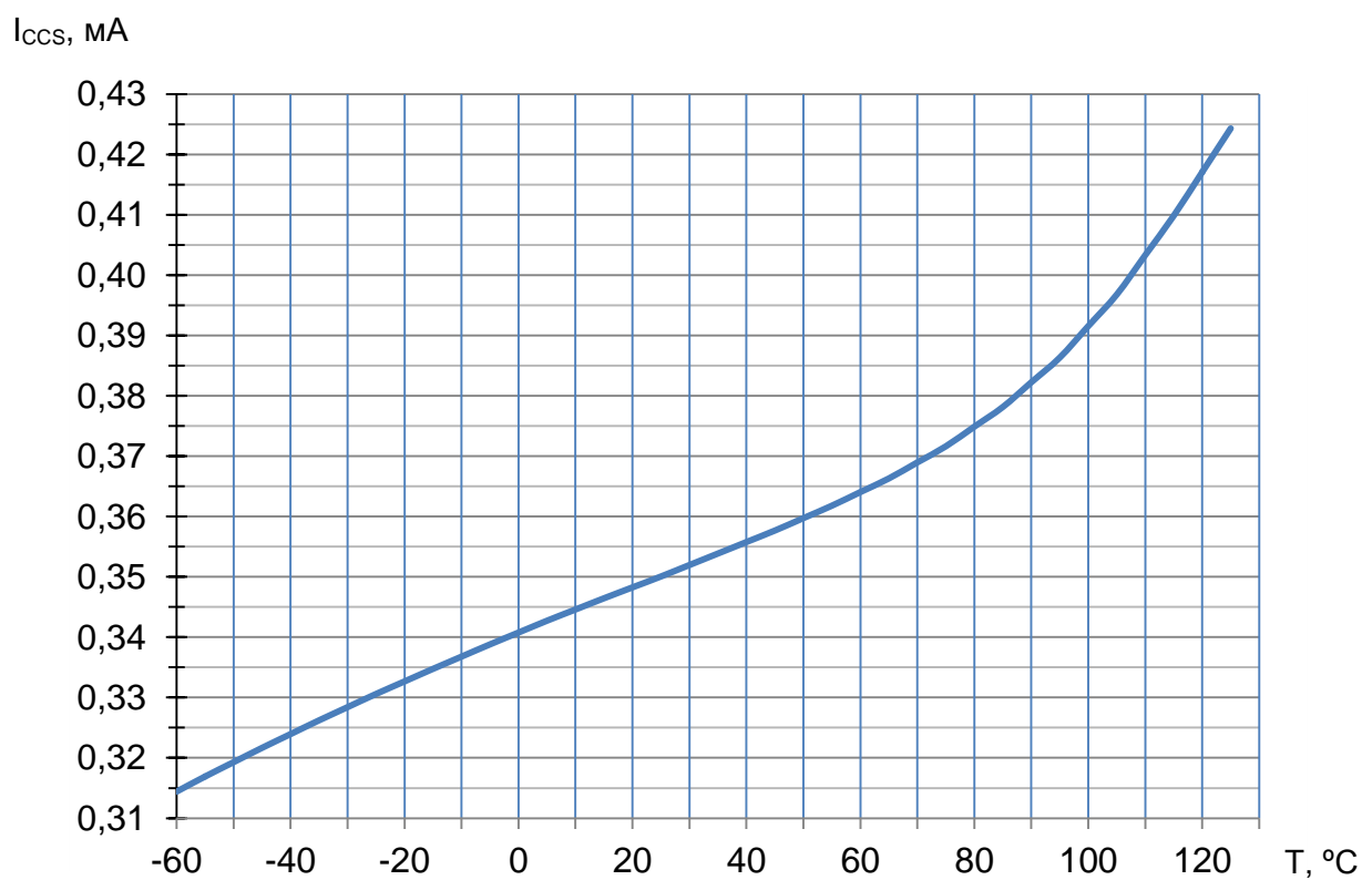
Рисунок 38 – Зависимость тока потребления в режиме хранения от температуры при U_{in} = 3,6\text{ V}
