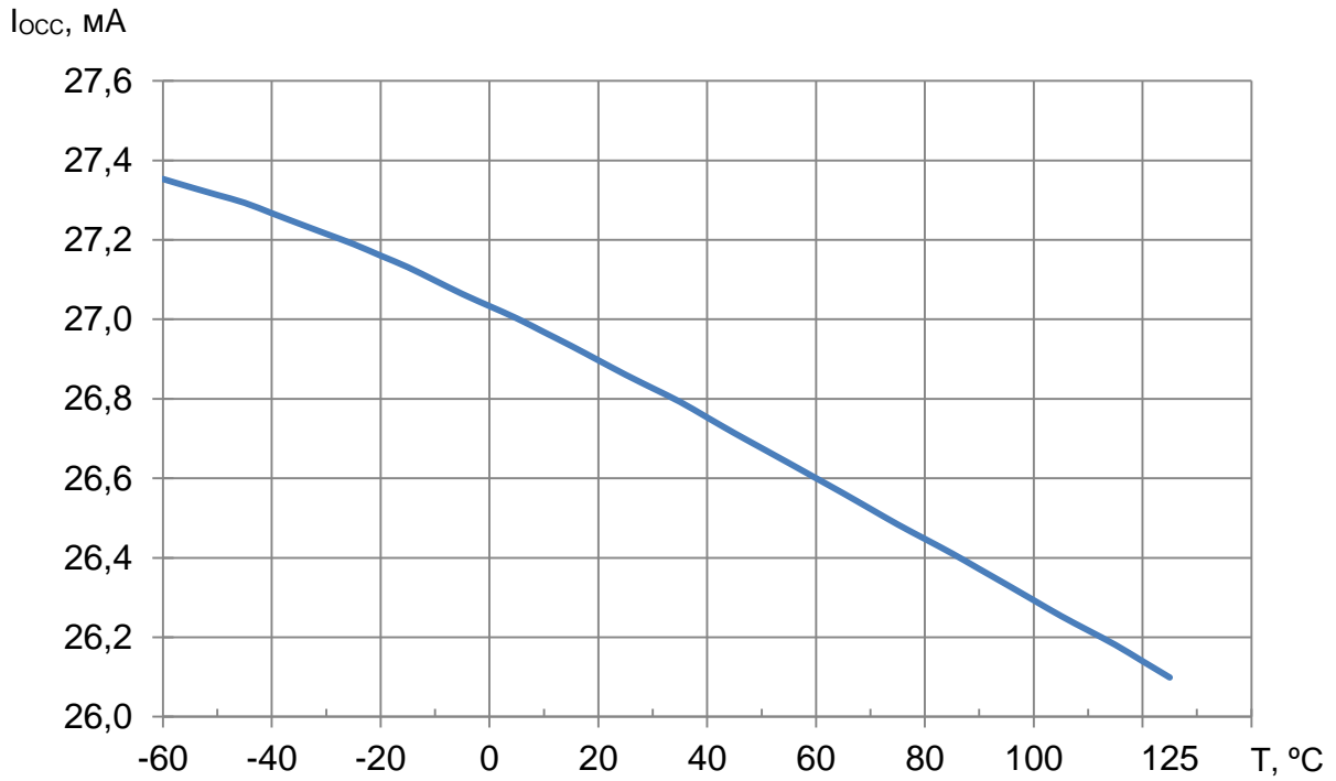
Рисунок 43 – Зависимость динамического тока потребления от температуры для при U_{CC} = 3,6 В, t_{CYR} = 65 нс
