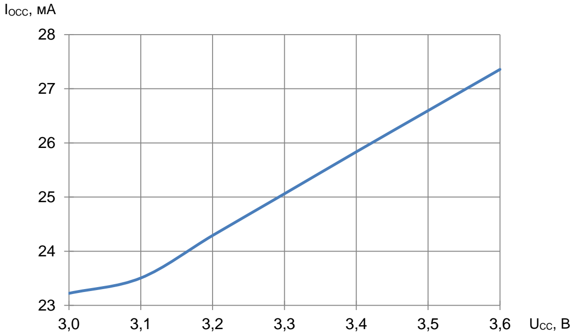
Рисунок 45 – Зависимость динамического тока потребления от напряжения питания при t_{CYR} = 65 нс, T = -60 °С
