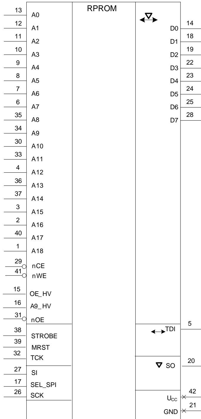
Рисунок 2 – Условно-графическое обозначение
