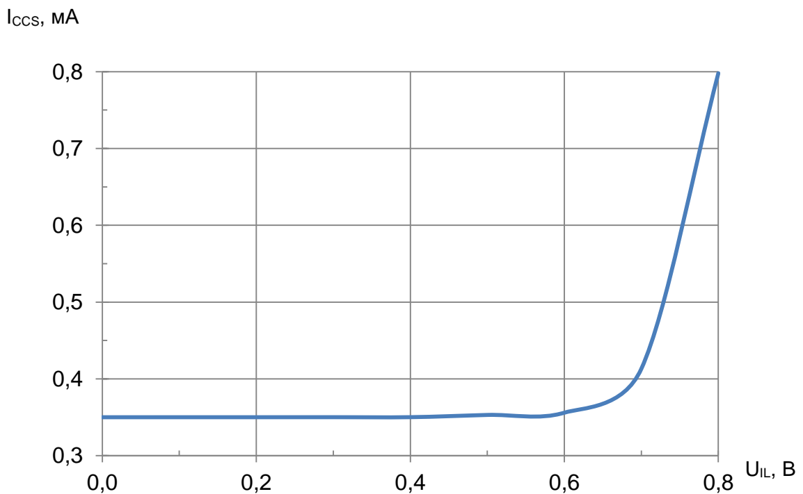
Рисунок 40 – Зависимость тока потребления в режиме хранения от входного напряжения низкого уровня при U_{CC} = 3,6 В, U_{IH} = 3,6 В, f = 0 МГц, T = 25 °С
