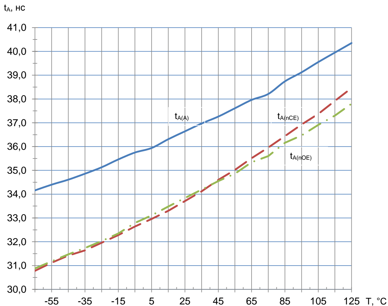
Рисунок 47 – Зависимость времени выборки адреса, t_{A(A)} , времени выборки по сигналу nCE , t_{A(nCE)} , времени выборки по сигналу nOE , t_{A(nOE)} от температуры при U_{CC} = 3,0 \text{ В}
