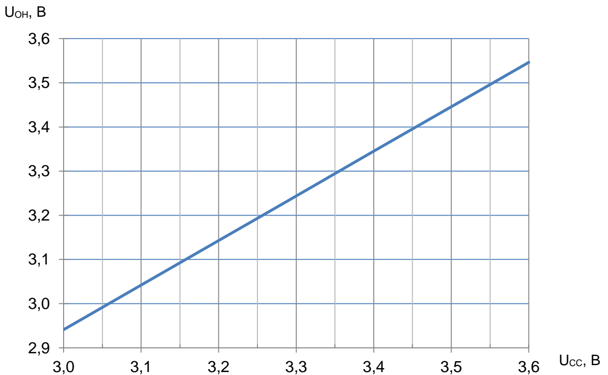
Рисунок 42 – Зависимость выходного напряжения высокого уровня от напряжения питания при I_{OH} = \text{минус } 2 мА, T = 25 °С
