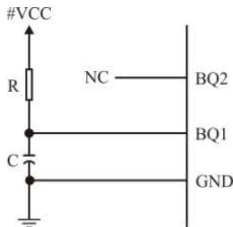
Рисунок 3.21 – Схема подключения внешней задающей RC-цепи
