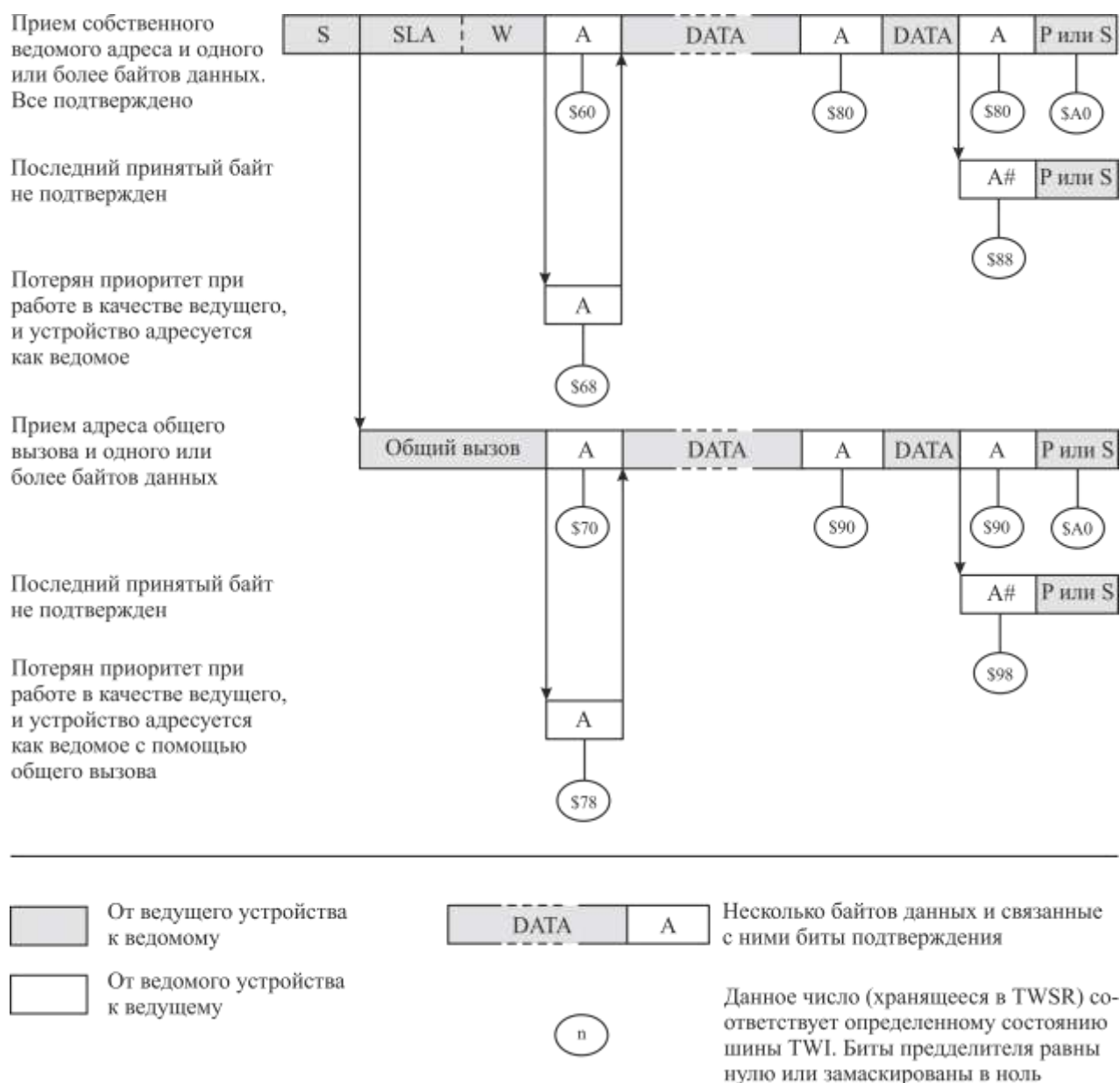
Рисунок 3.102 – Форматы и состояния в режиме ведомого приемника
