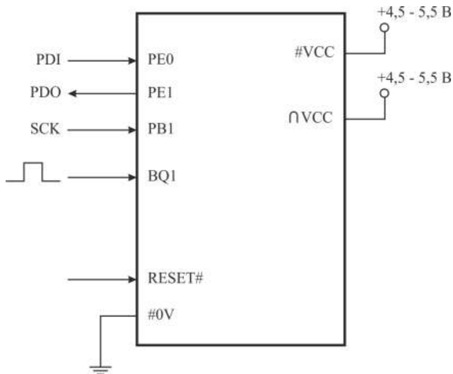
Рисунок 3.145 – Сигналы последовательного программирования
