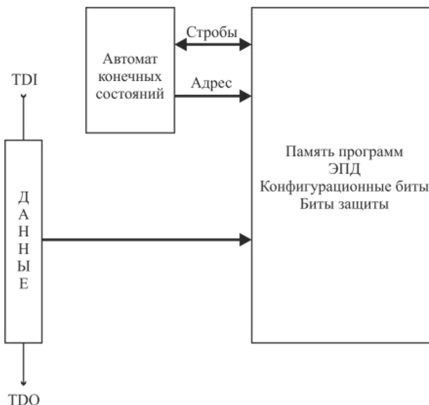
Рисунок 3.151 – Виртуальный регистр загрузки страницы памяти программ
