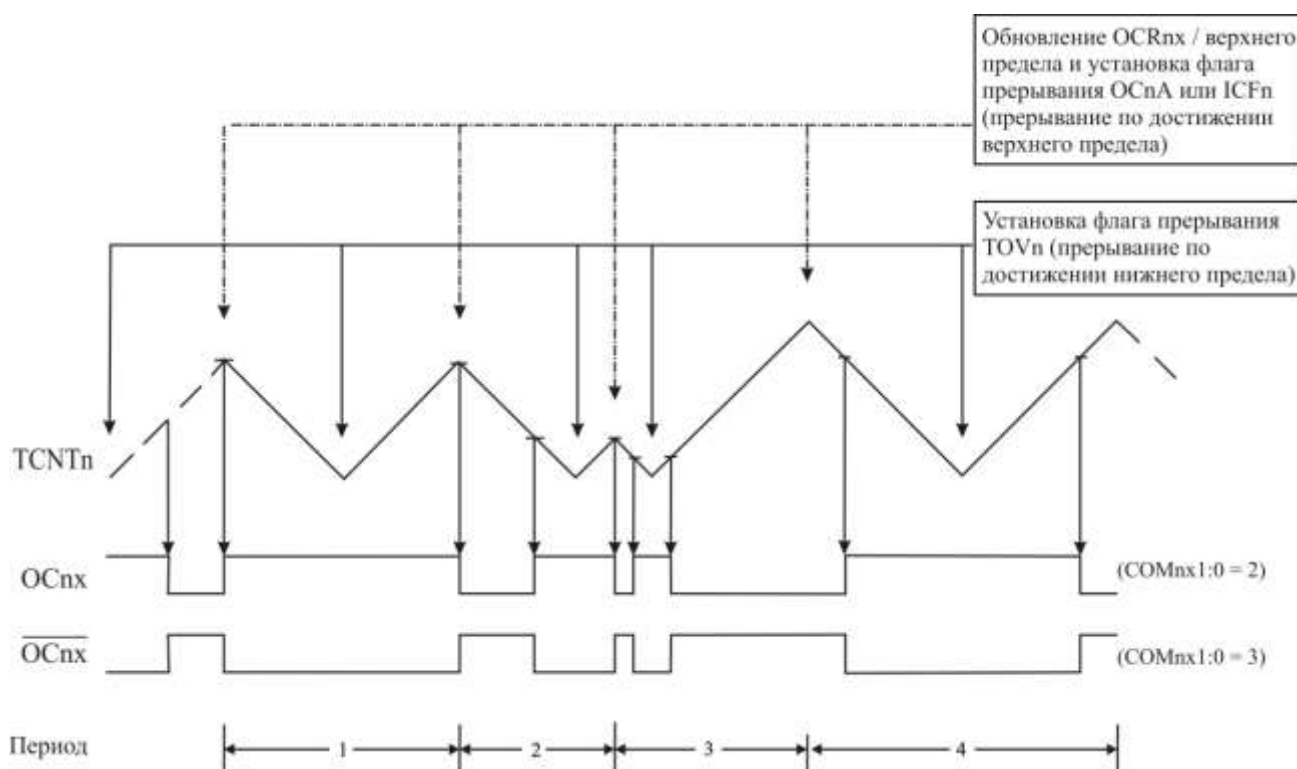
Рисунок 3.54 – Временная диаграмма для режима ШИМ с фазовой коррекцией
