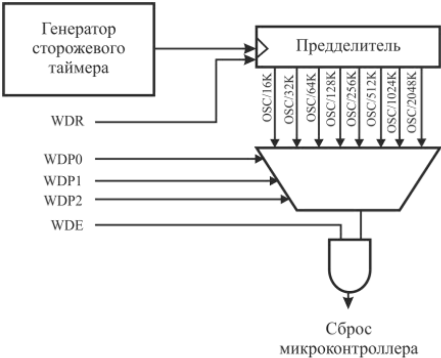
Рисунок 3.29 – Сторожевой таймер
