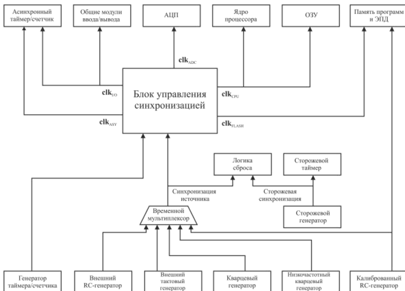
Рисунок 3.19 – Распределение тактовых сигналов
