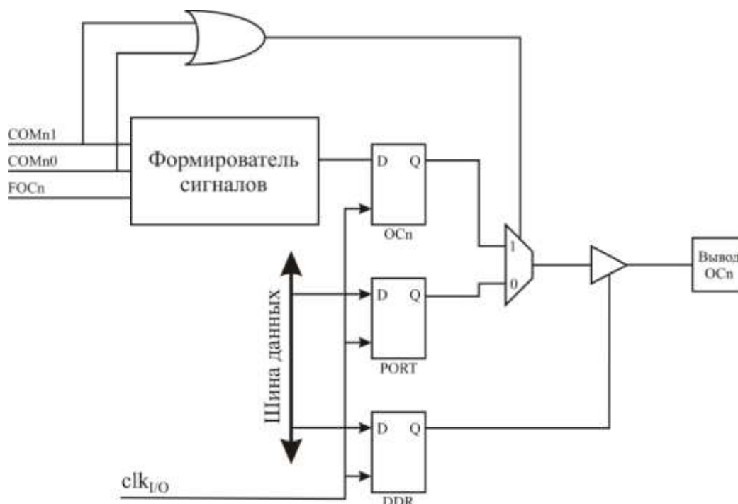
Рисунок 3.38 – Схема блока формирования выходного сигнала
