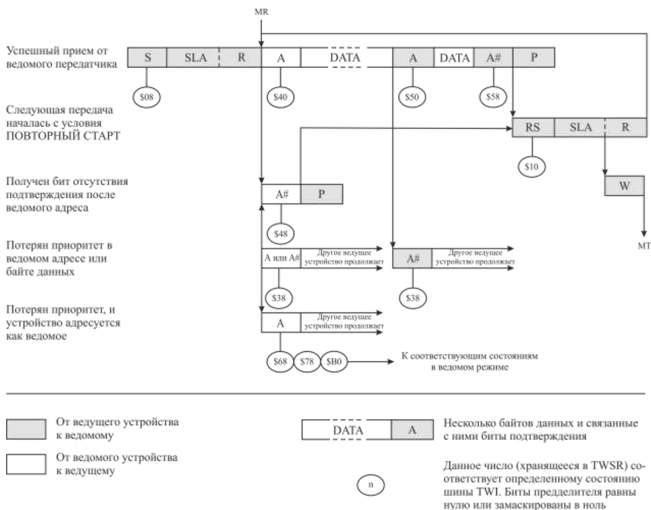
Рисунок 3.100 – Форматы и состояния в режиме ведущего приемника
