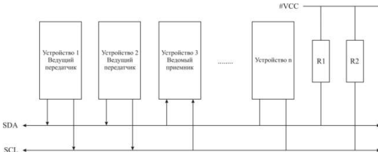
Рисунок 3.106 – Пример арбитража
