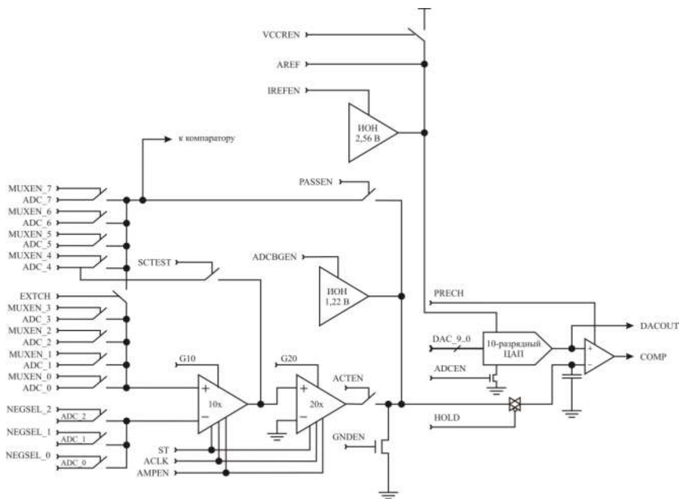
Рисунок 3.132 – Аналого-цифровой преобразователь
