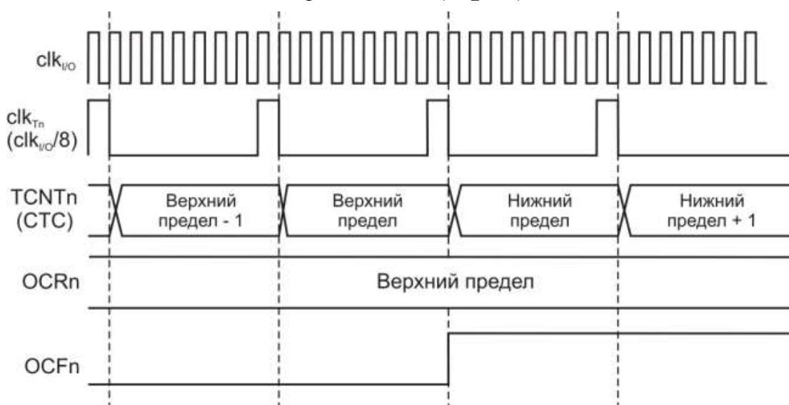
Рисунок 3.44 – Временная диаграмма таймера/счетчика, установка флага OCF0, с делением ( f_{\text{clk\_I/O}}/8 )
