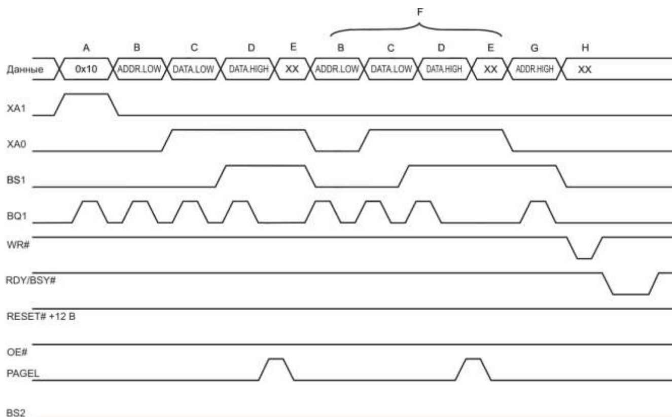
Рисунок 3.138 – Временная диаграмма программирования памяти программ
