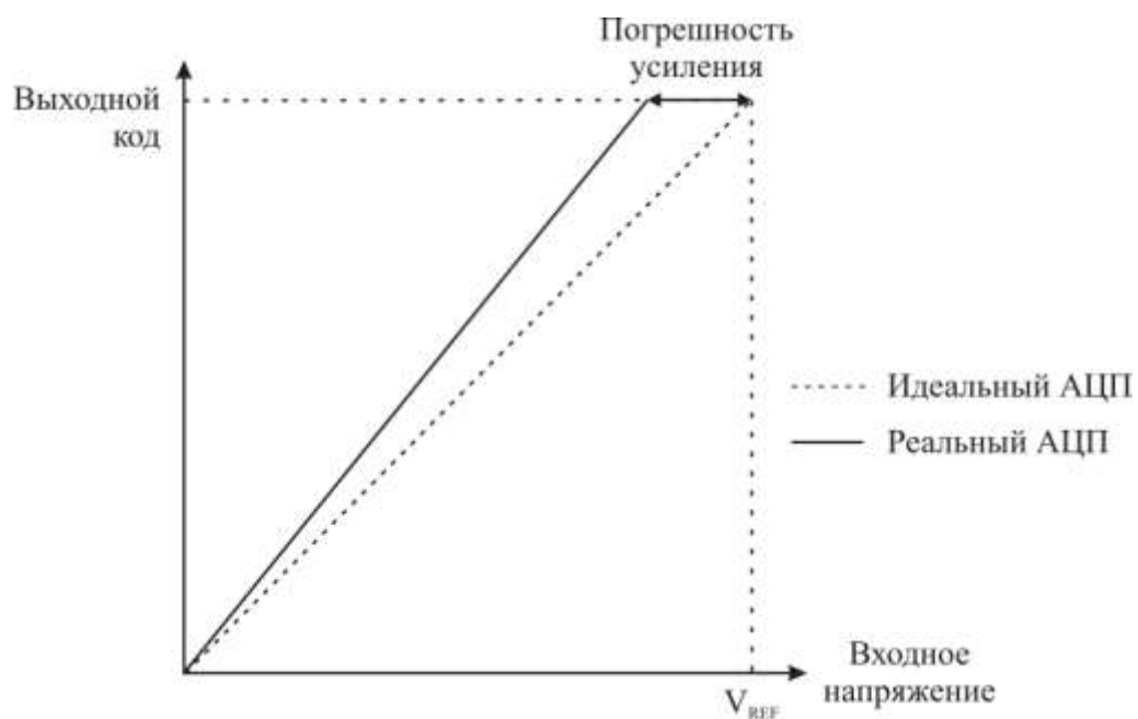
Рисунок 3.117 – Погрешность усиления
