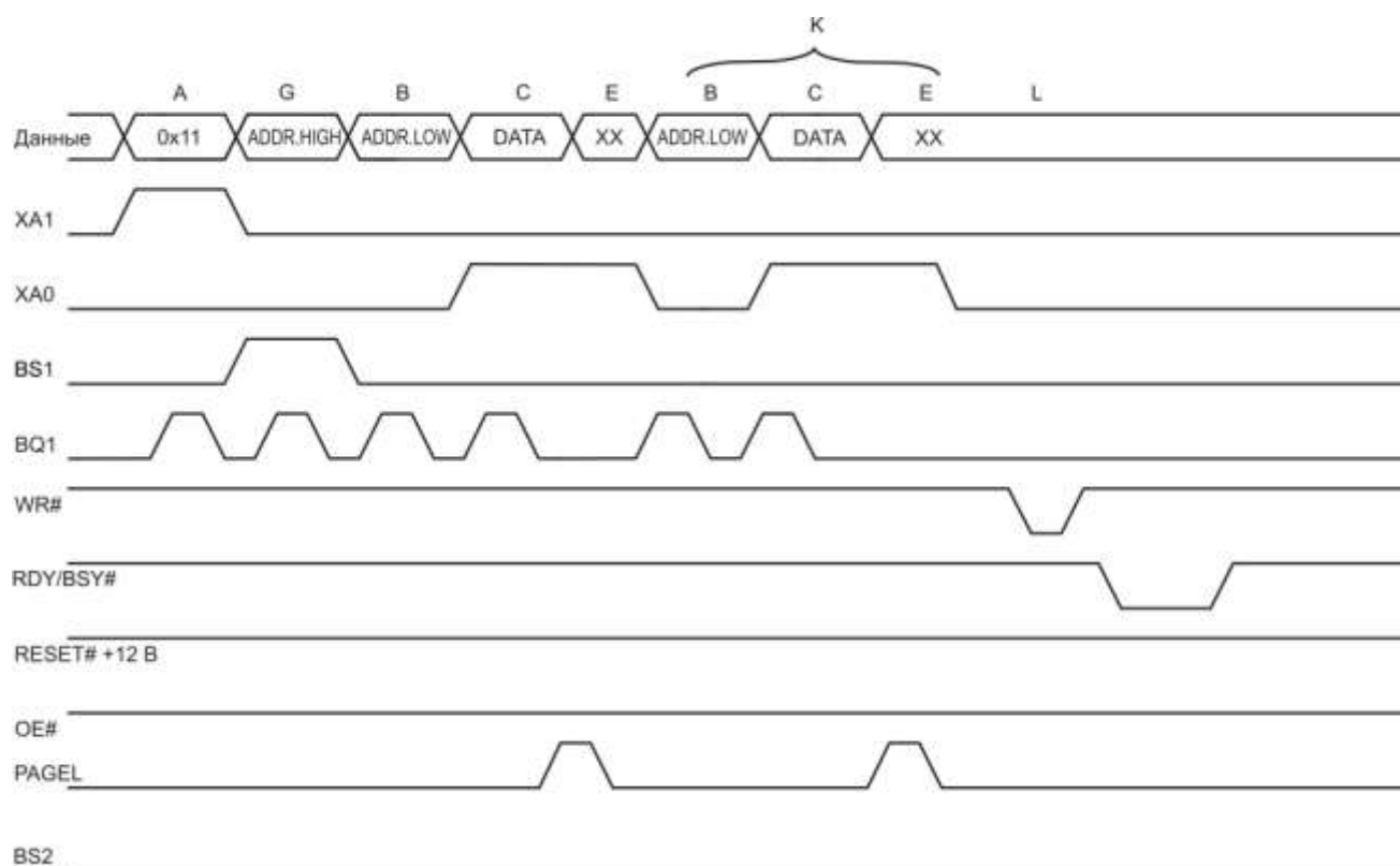
Рисунок 3.139 – Временная диаграмма программирования ЭПД
