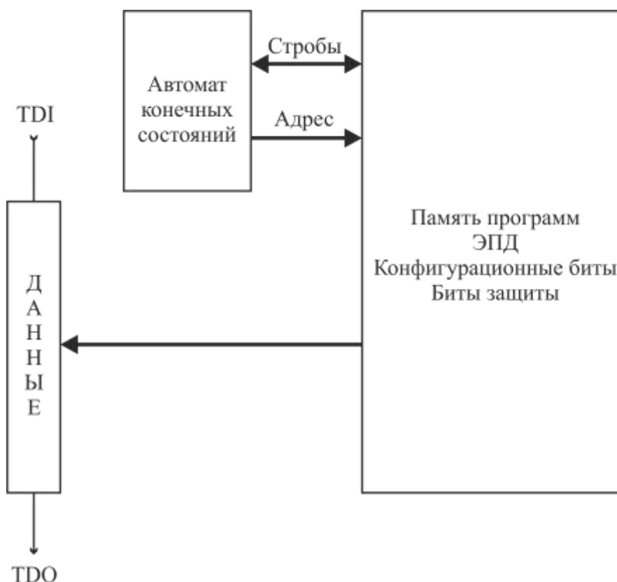
Рисунок 3.152 – Виртуальный регистр чтения страницы памяти программ
