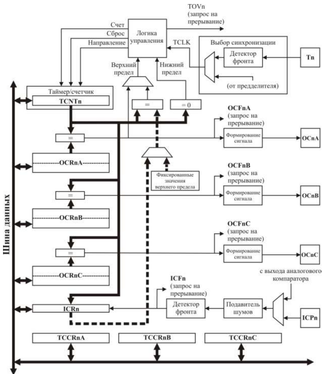
Рисунок 3.47 – Структурная схема 16-разрядного таймера/счетчика
