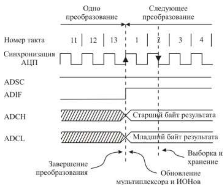
Рисунок 3.113 – Временная диаграмма работы АЦП в автономном режиме
