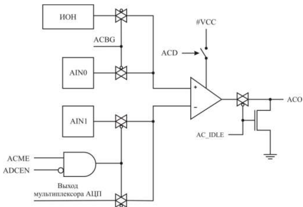
Рисунок 3.130 – Аналоговый компаратор
