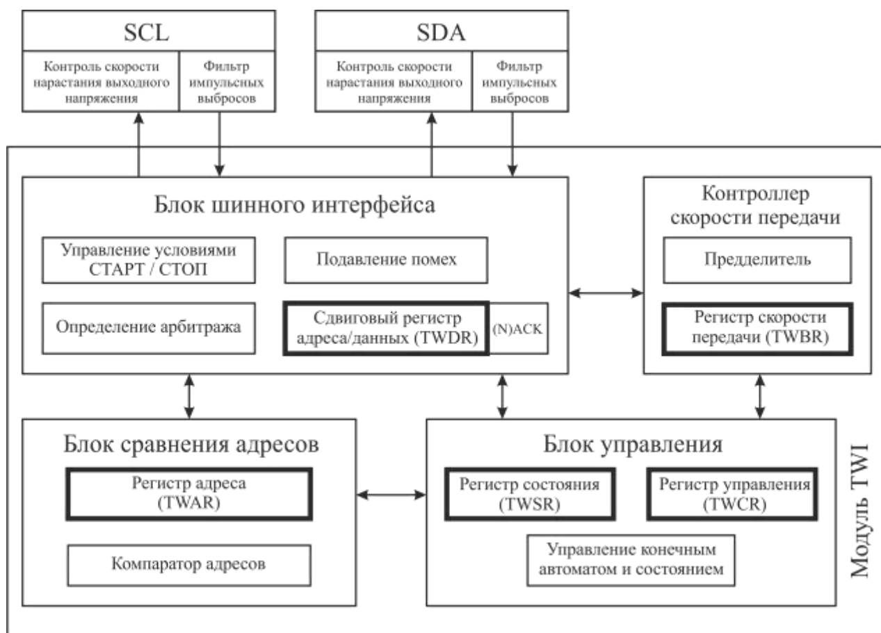
Рисунок 3.95 – Структурная схема модуля TWI
