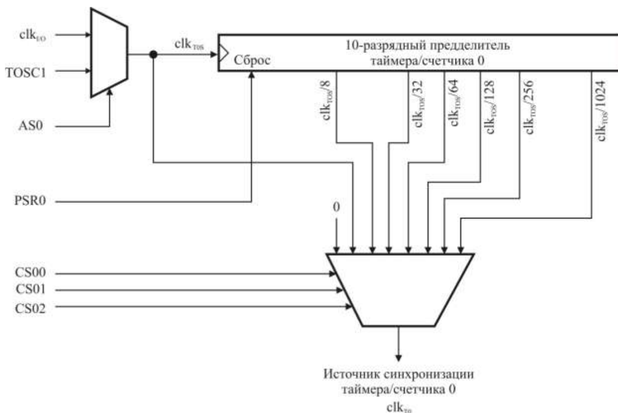
Рисунок 3.46 – Предделитель таймера/счетчика 0
