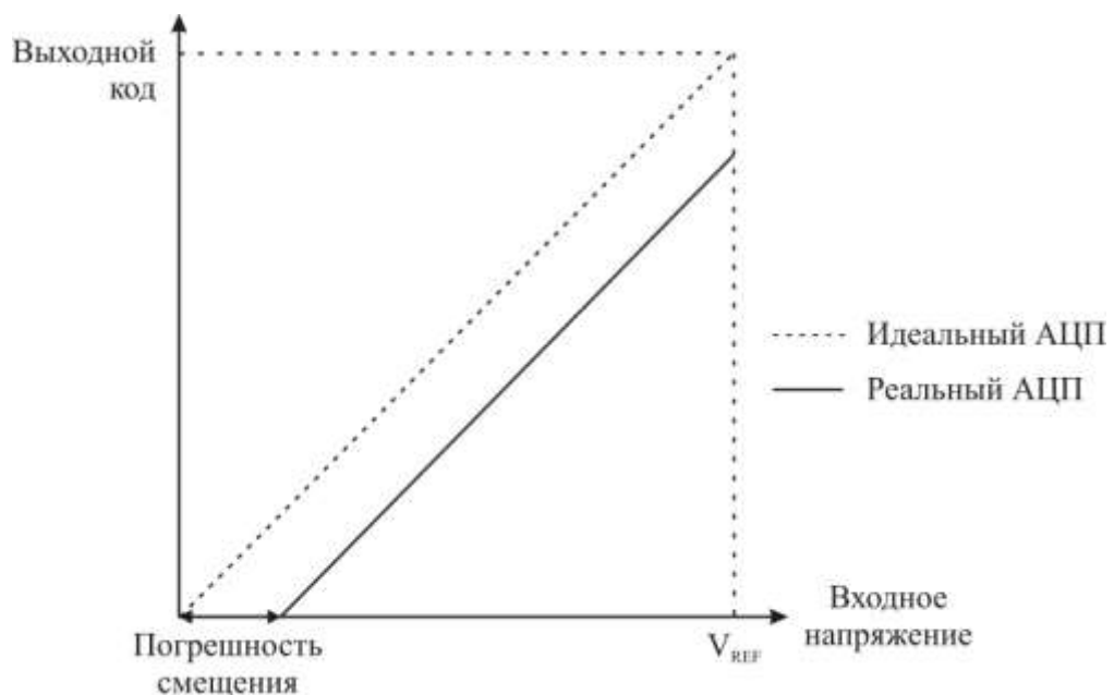
Рисунок 3.116 – Погрешность смещения
