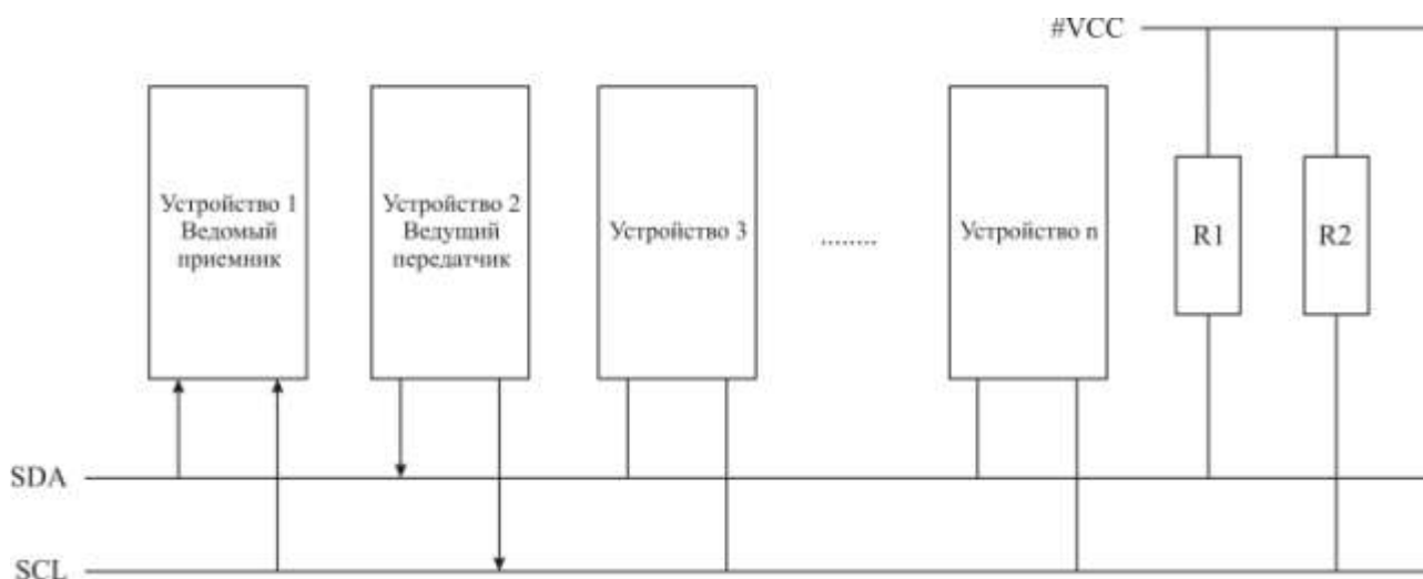
Рисунок 3.101 – Передача данных в режиме ведомого приемника
