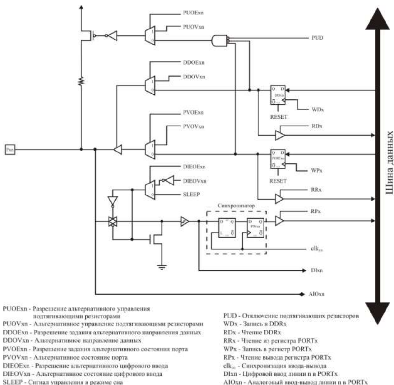
Рисунок 3.34 – Альтернативные функции порта
