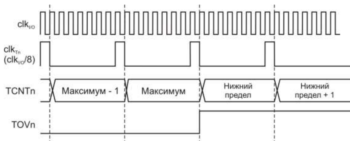
Рисунок 3.43 – Временная диаграмма таймера/счетчика с делением ( f_{\text{clk\_I/O}}/8 )
