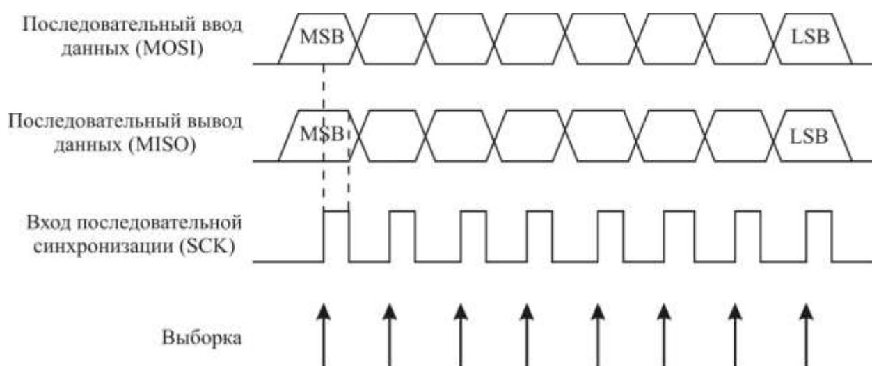
Рисунок 3.146 – Временная диаграмма сигналов при последовательном программировании через SPI
