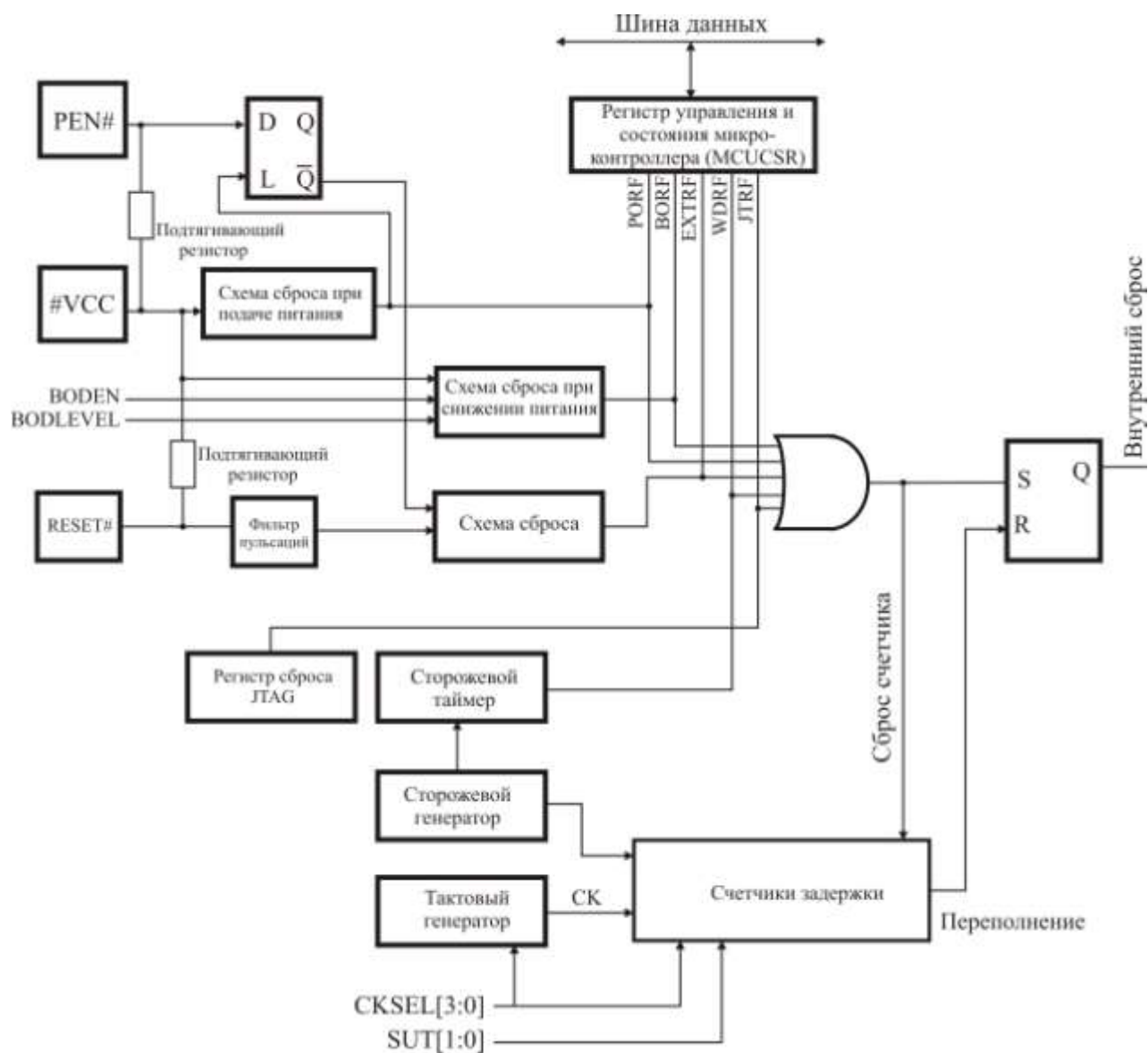
Рисунок 3.23 – Логика сброса
