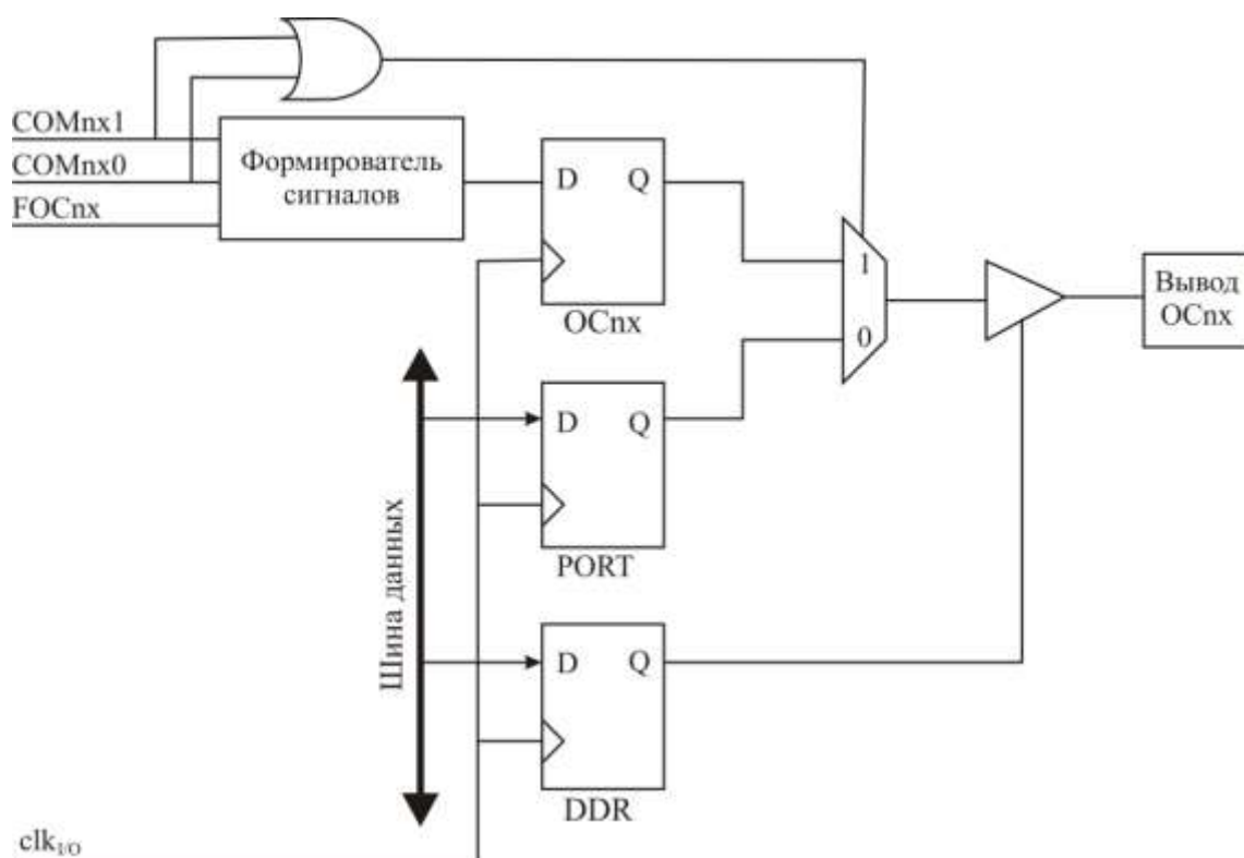
Рисунок 3.51 – Схема блока формирования выходного сигнала
