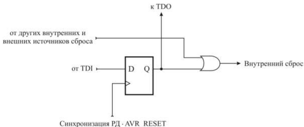
Рисунок 3.124 – Регистр сброса
