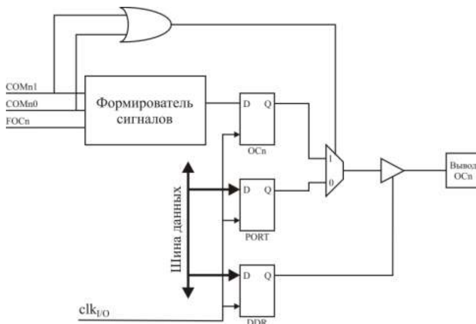
Рисунок 3.65 – Схема блока формирования выходного сигнала
