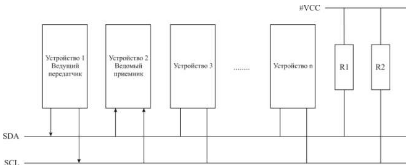
Рисунок 3.97 – Передача данных в режиме ведущего передатчика
