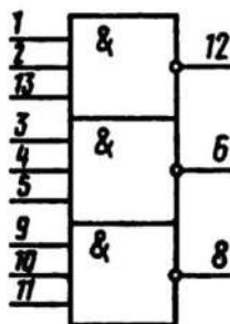
Условное графическое обозначение КР530ЛА4
