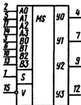
Условное графическое обозначение К533КП16, КМ533КП16
