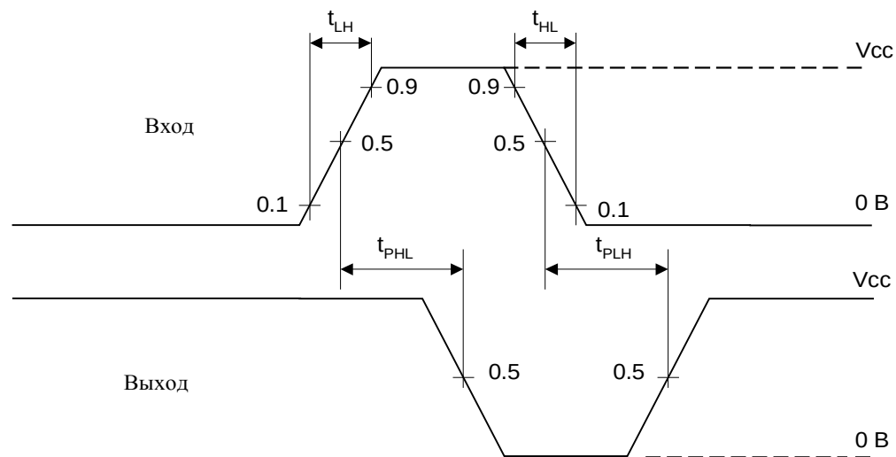
Временная диаграмма
