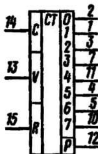
Условное графическое обозначение К564ИЕ9, КФ564ИЕ9В
