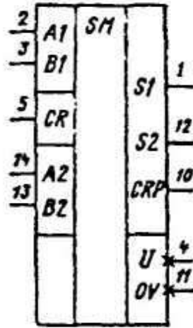
Условное графическое обозначение К13ЗИМ2
