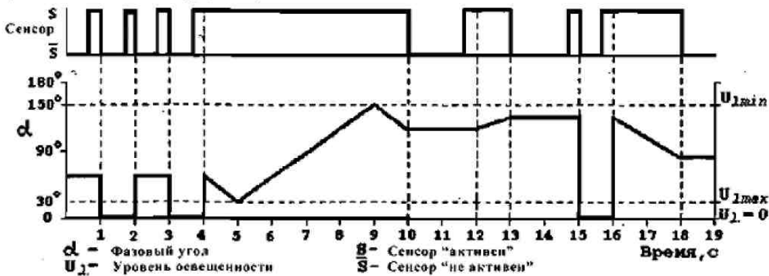
Рис 2. Временные диаграммы работы
