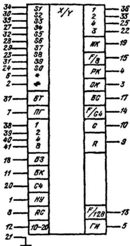
Условное графическое обозначение К145ИК8
