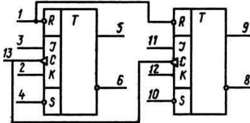
Условное графическое обозначение К530ТВ11
