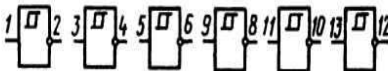
Условное графическое обозначение К533ТЛ2
